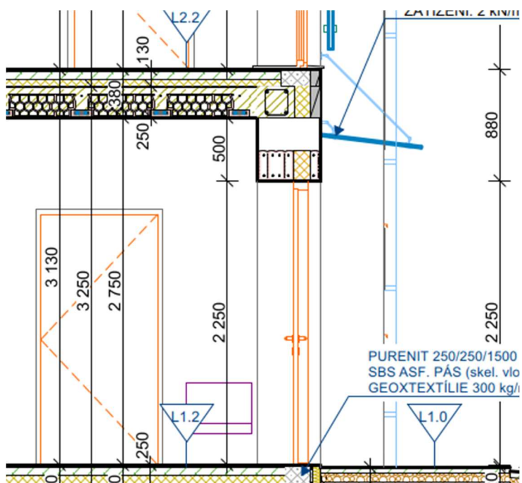
Obrázek 1: Chyba - nejasnost kóty (Zdroj – projektová dokumentace „ŘEZ A-A“)
