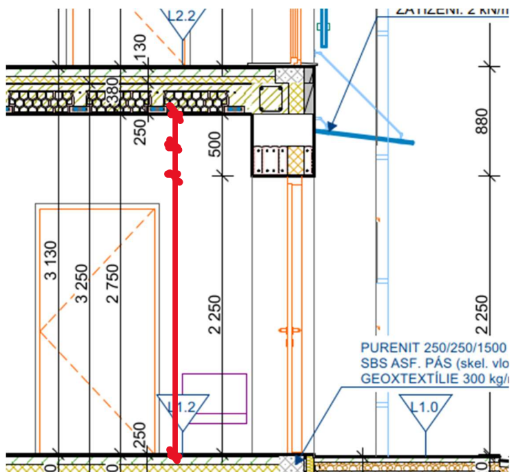
Obrázek 2: Oprava - nejasnost kóty (Zdroj – projektová dokumentace „ŘEZ A-A“)
