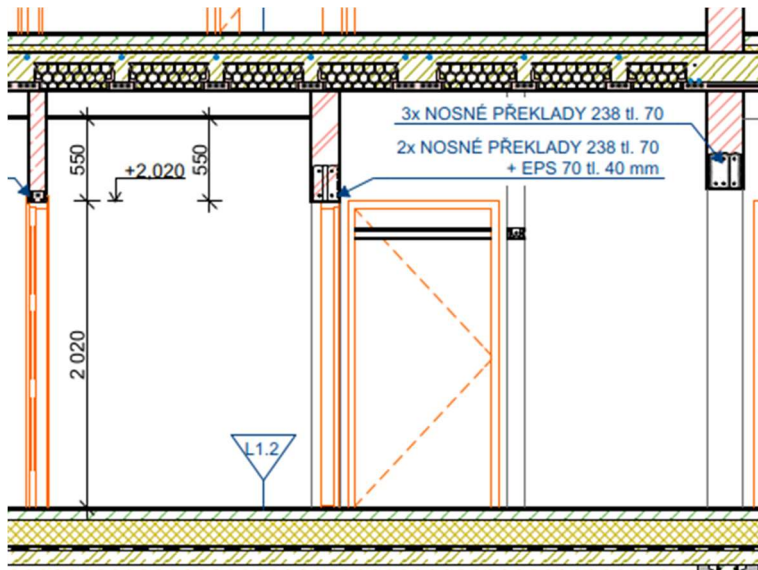
Obrázek 3: Chyba - Stěna v řezu (Zdroj – projektová dokumentace „ŘEZ B-B“)
