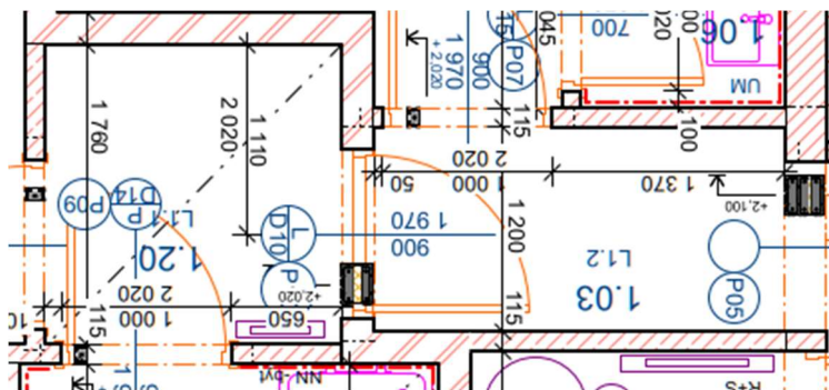
Obrázek 4: Chyba - Stěna v půdorysu (Zdroj – projektová dokumentace „Půdorys 1.NP“)
