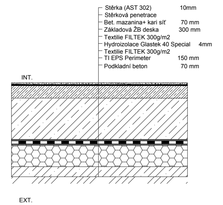
P01-SKLADBA PODLAHY NA TERÉNU (1.NP)
