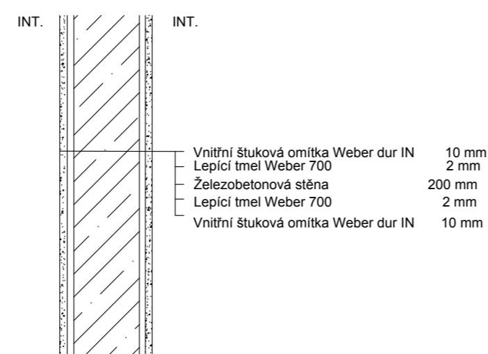
ST03 - SKLADBA VNITŘNÍ NOSNÉ STĚNY
