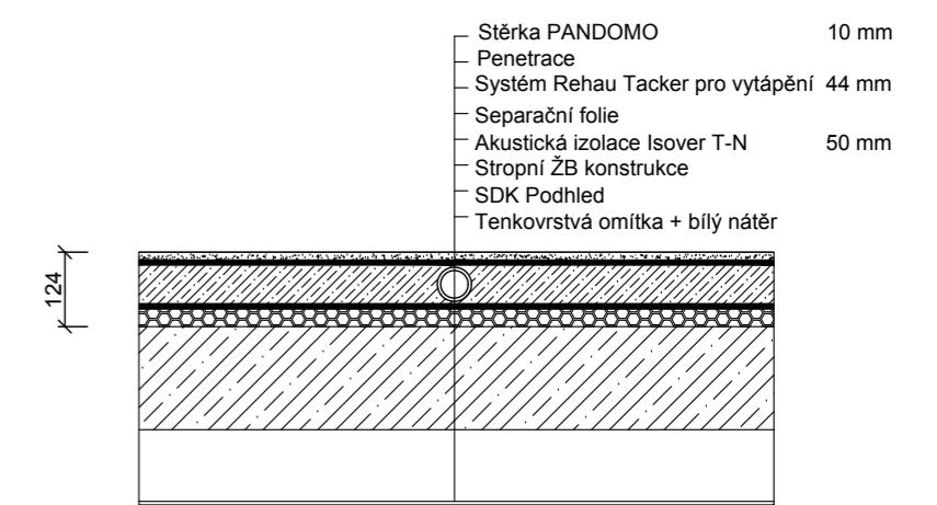
P05-SKLADBA PODLAHY 2.NP
