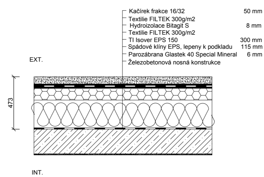
S03-SKLADBA STŘECHY NAD 6.NP (ŽB NOSNÁ KCE)
