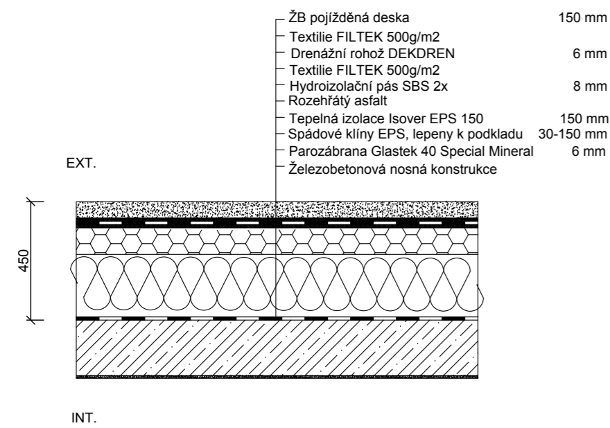
S01-SKLADBA STŘECHY NAD 1.PP (POJÍŽDĚNÁ)
