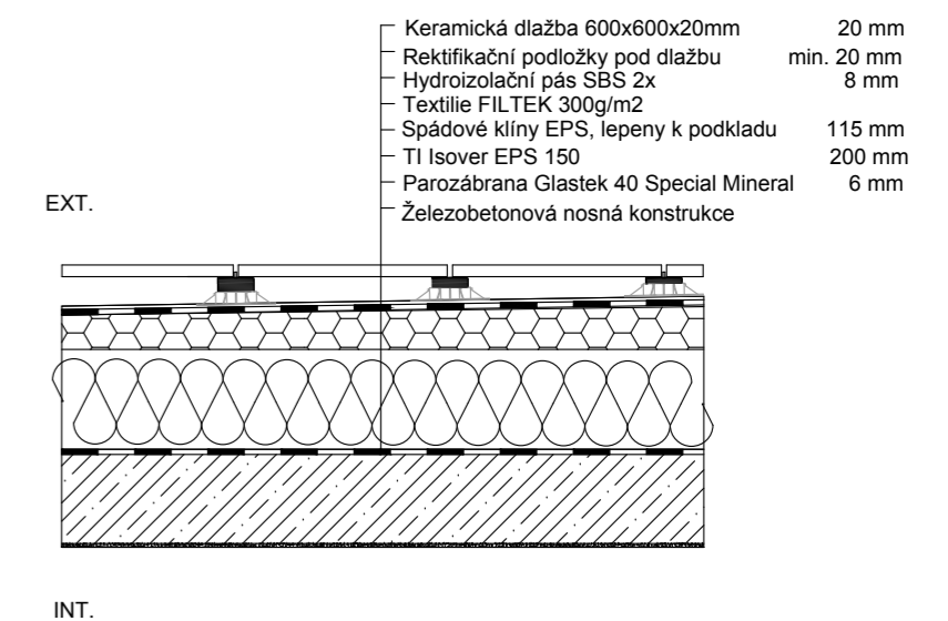
P06-SKLADBA PODLAHY (LODŽIE)
