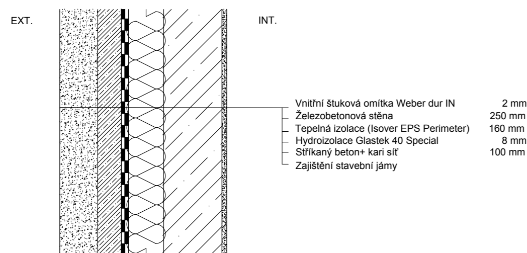
ST01 - SKLADBY NOSNÉ STĚNY 1.PP (černá vana)
