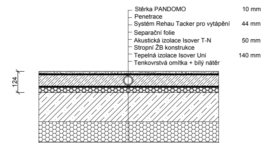
P04-SKLADBA PODLAHY NAD GARÁŽÍ (KOMERČNÍ PLOCHY)
