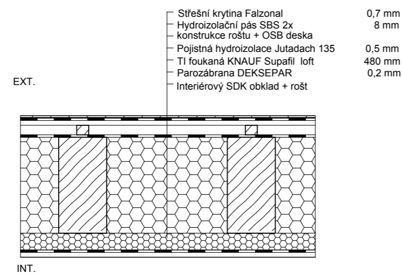
S02-SKLADBA STŘECHY NAD 2.NP a 6.NP (DŘEVĚNÉ NOSNÁ KCE)
