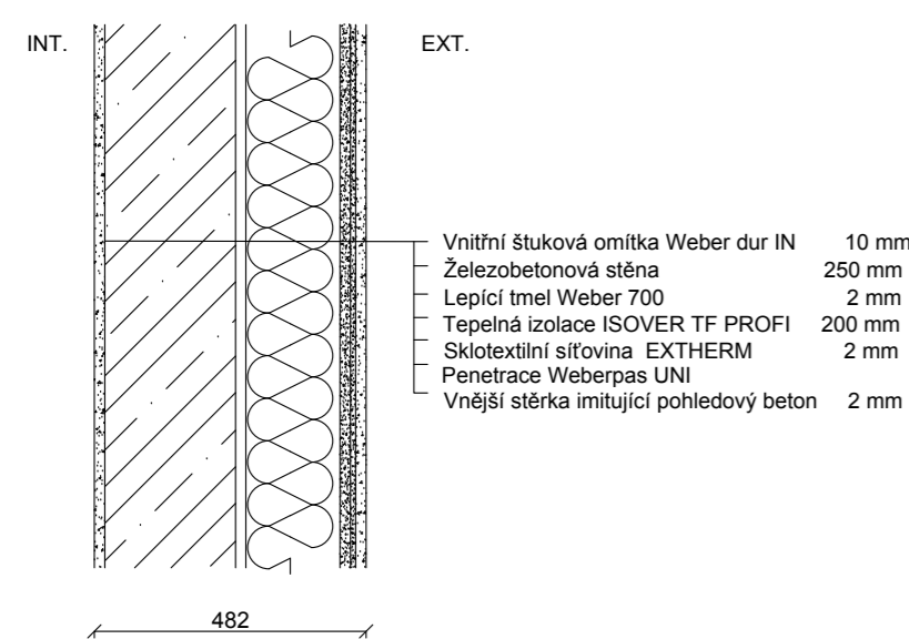
ST02 - SKLADBA OBVODOVÉ STĚNY
