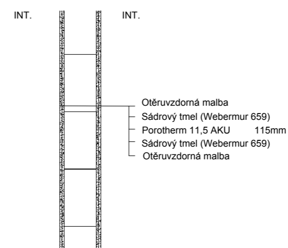
PR01-SKLADBA PŘÍČKY
