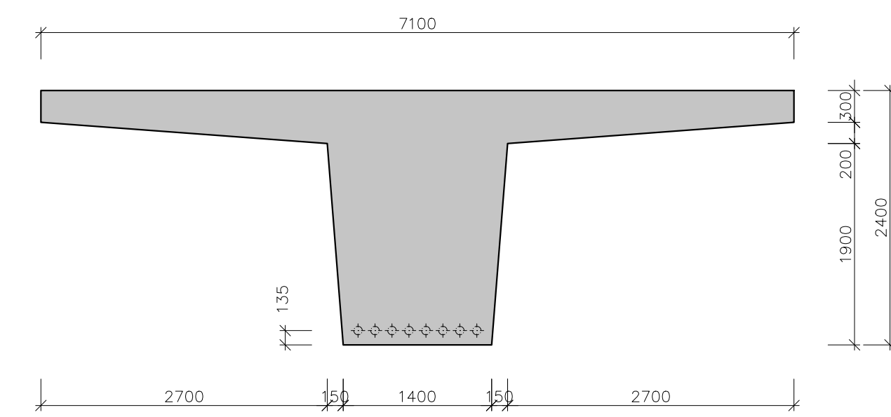
ŘEZ V POLI P2–P3 1:50
