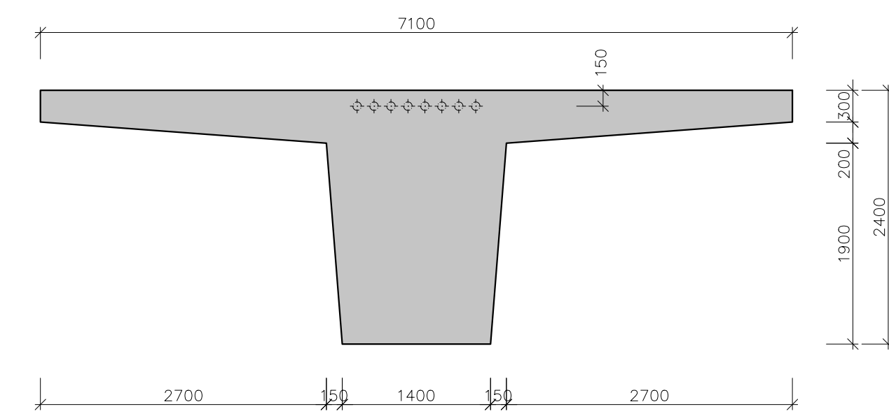
ŘEZ NAD PODPOROU P3 1:50
