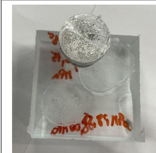
Lepidlo Loctite EA 9455, předúprava odmaštěním, druhé odtrhy
