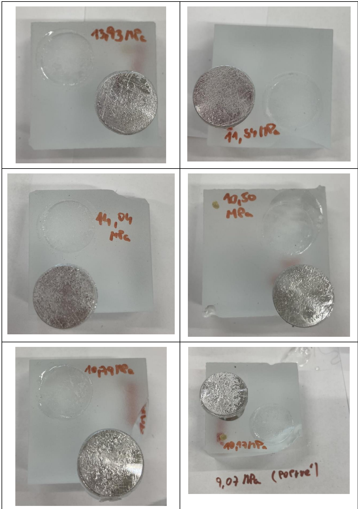
Lepidlo Loctite EA 9455, předúprava tryskáním, první odtrhy
