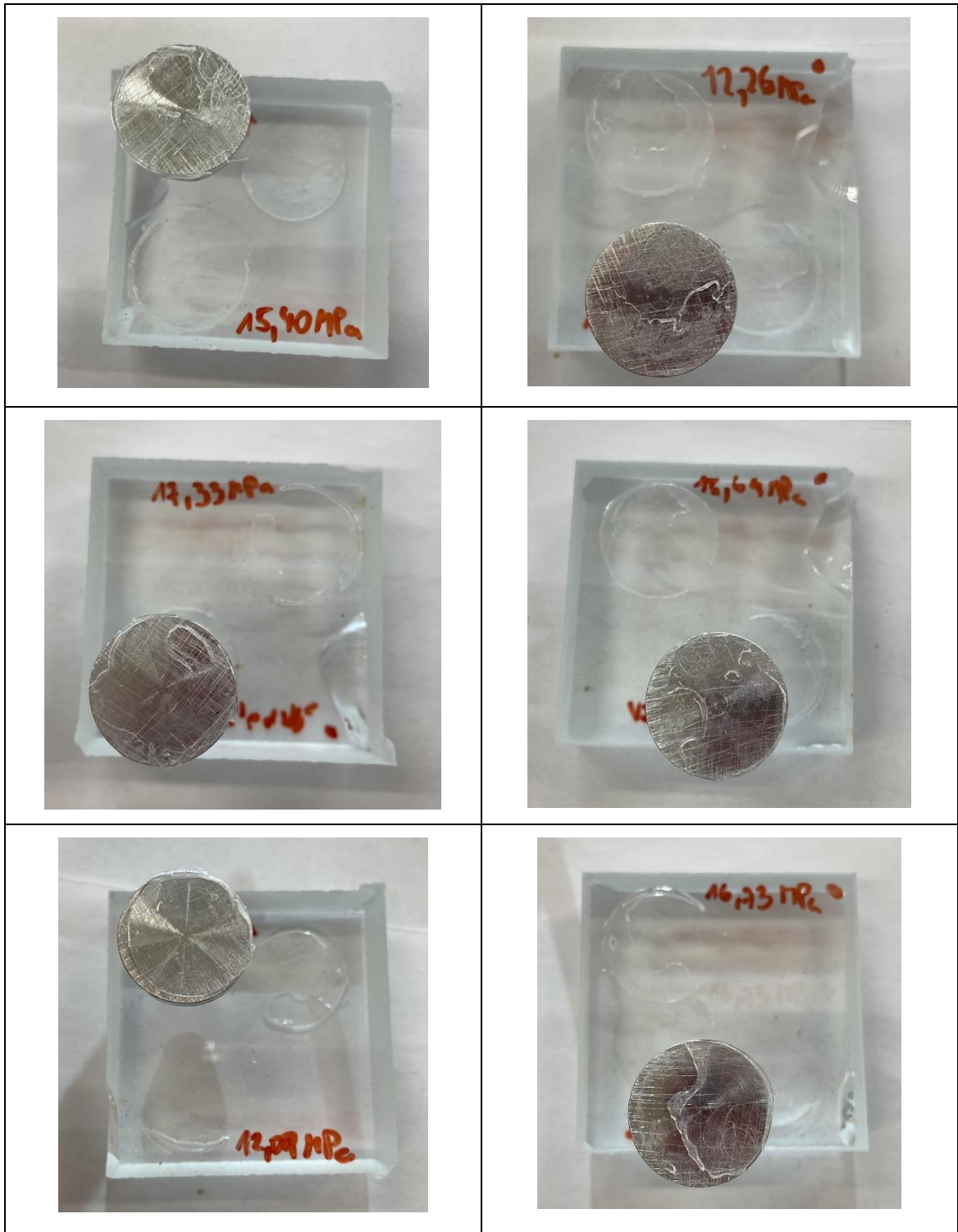
Lepidlo Auratech AR 708, předúprava odmaštěním, první odtrhy
