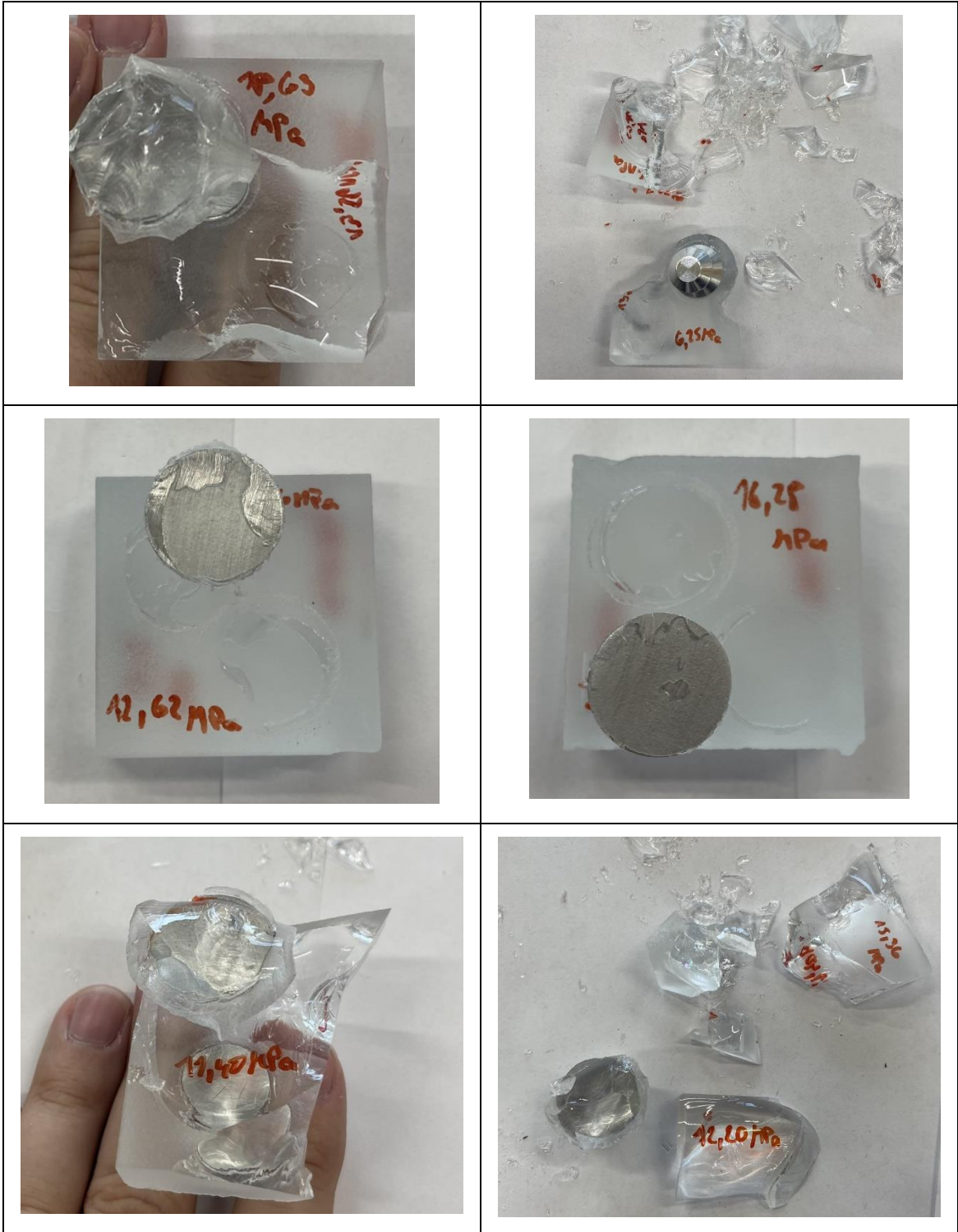
Lepidlo Auratech AR 708, předúprava tryskáním, druhé odtrhy
