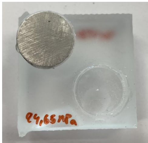
Lepidlo Loctite EA 9455, předúprava leptáním, první odtrhy
