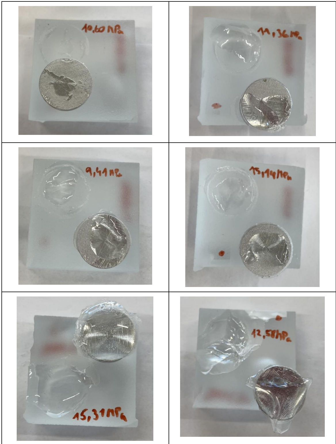
Lepidlo Auratech AR 011, předúprava tryskáním, první odtrhy
