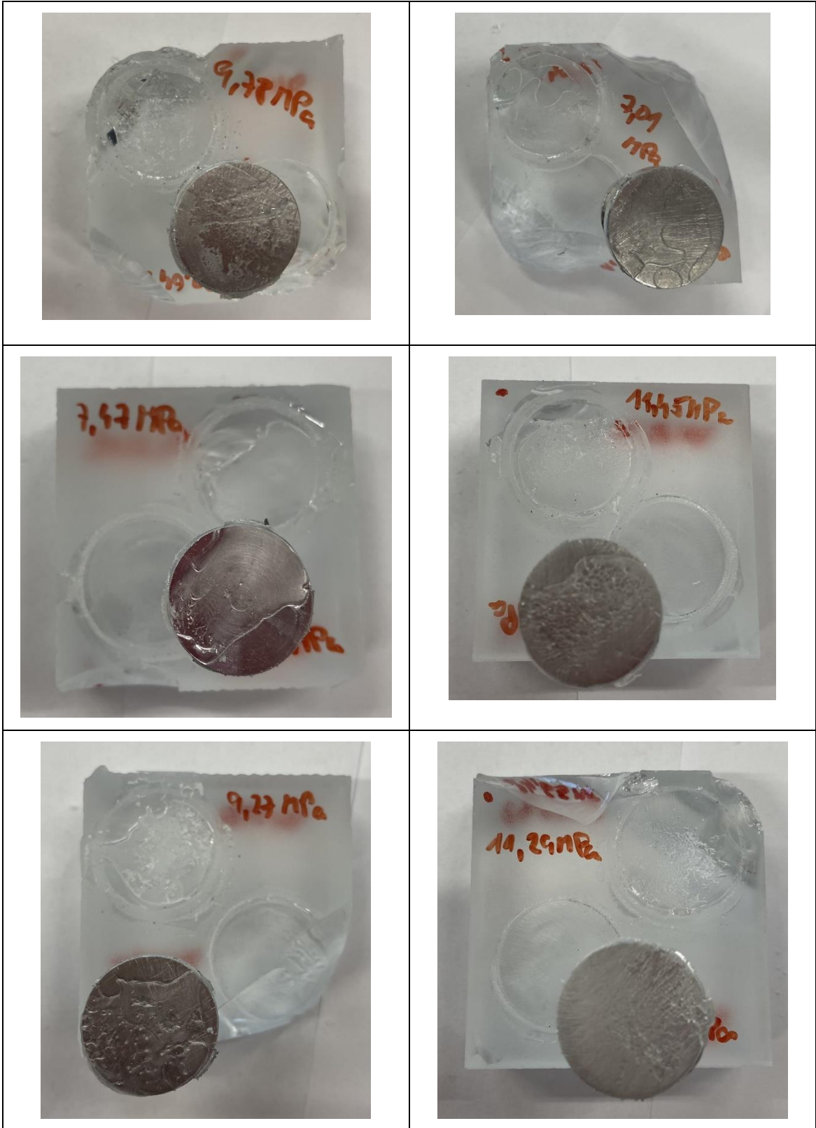
Lepidlo Loctite EA 9455, předúprava leptáním, druhé odtrhy
