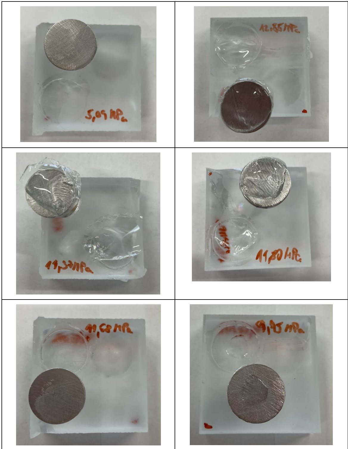
Lepidlo Auratech AR 011, předúprava leptáním, první odtrhy
