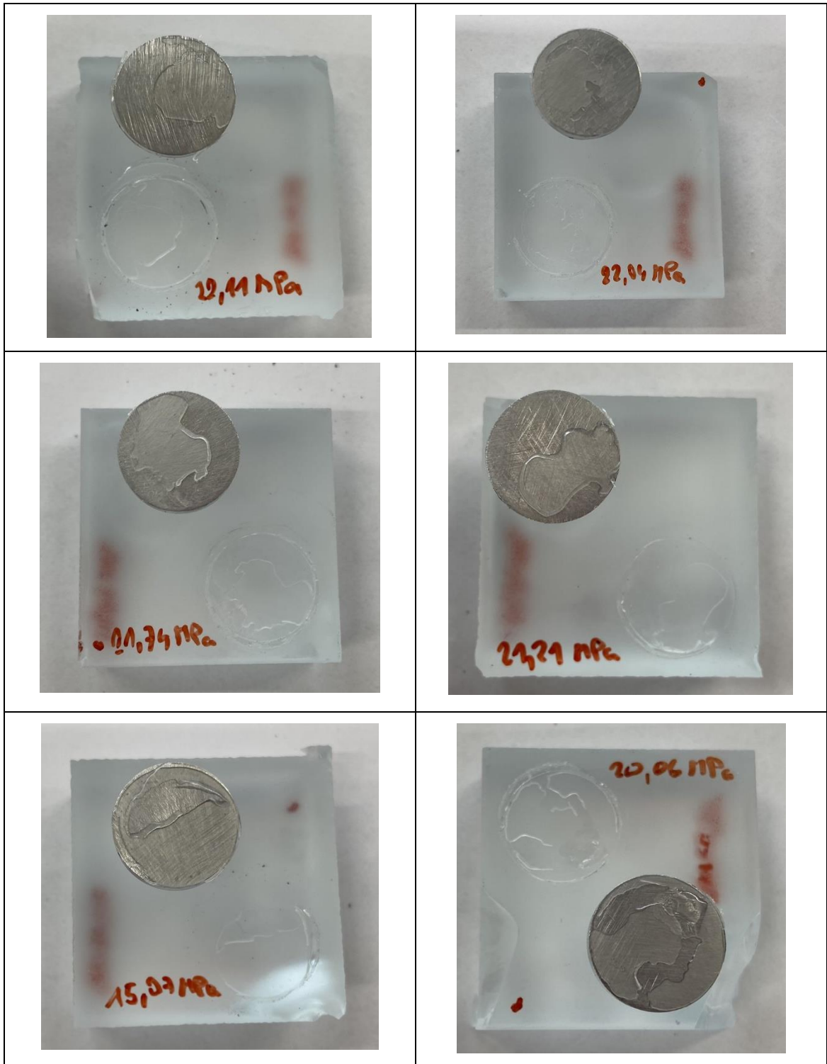
Lepidlo Auratech AR 708, předúprava leptáním, první odtrhy
