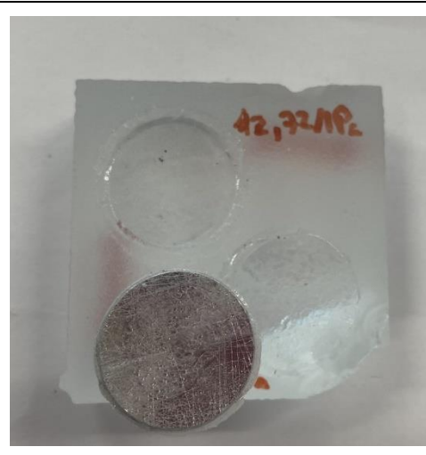
Lepidlo Loctite EA 9455, předúprava tryskáním, druhé odtrhy
