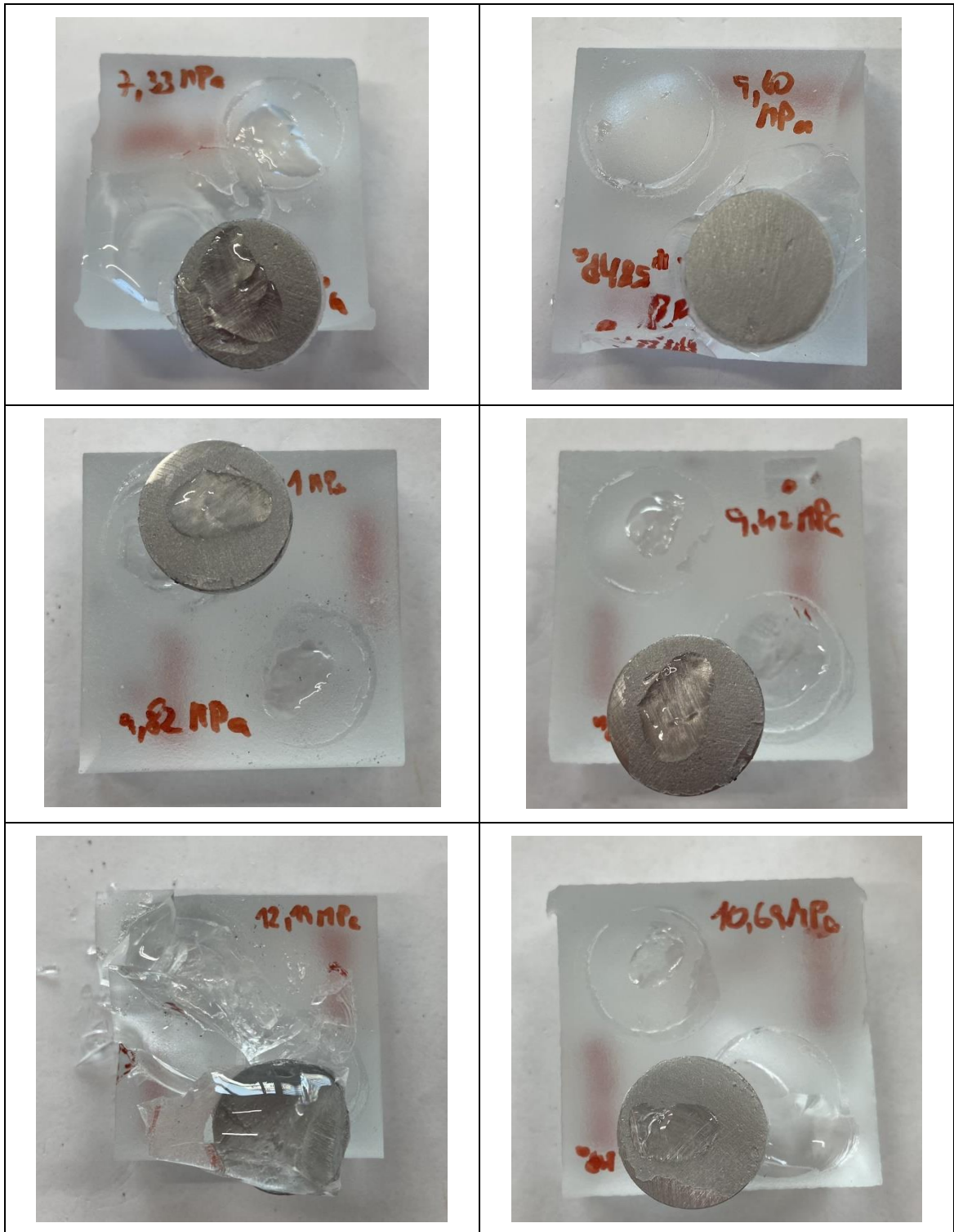
Lepidlo Auratech AR 011, předúprava tryskáním, druhé odtrhy
