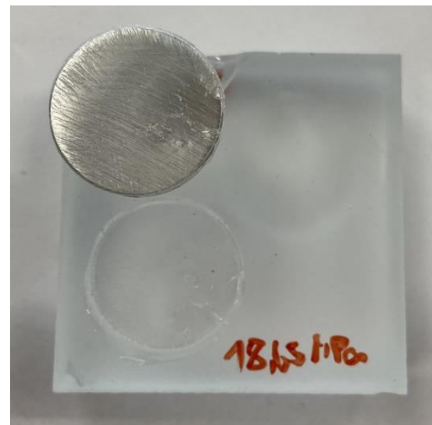
Lepidlo Loctite EA 9455, předúprava leptáním, první odtrhy
