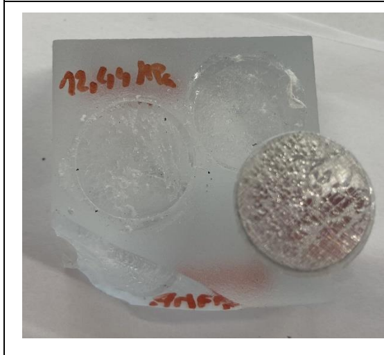
Lepidlo Loctite EA 9455, předúprava tryskáním, druhé odtrhy
