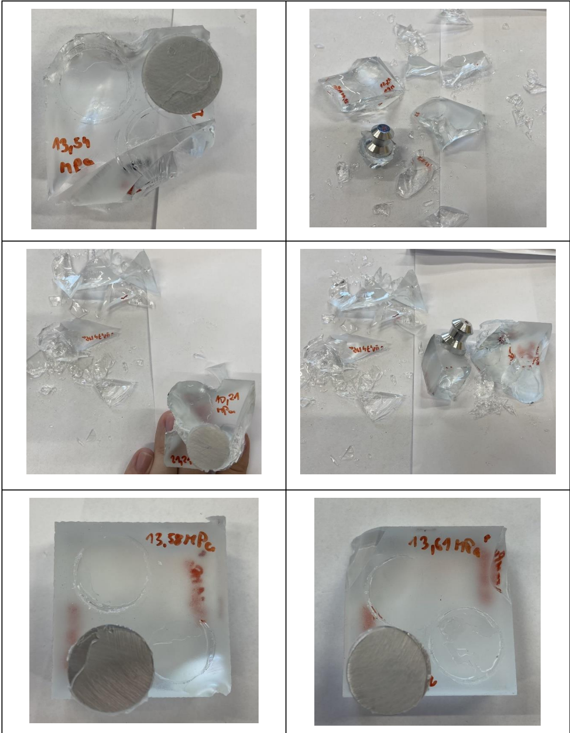
Lepidlo Auratech AR 708, předúprava leptáním, druhé odtrhy
