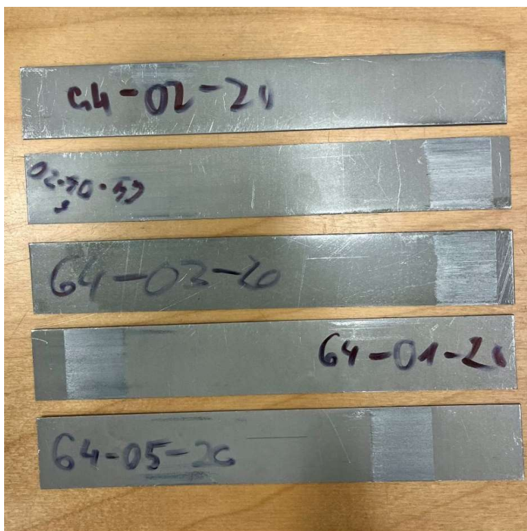
Obr. 1 – Vzorky tažené při 20 mm/min a 20 °C [Foto autor]
