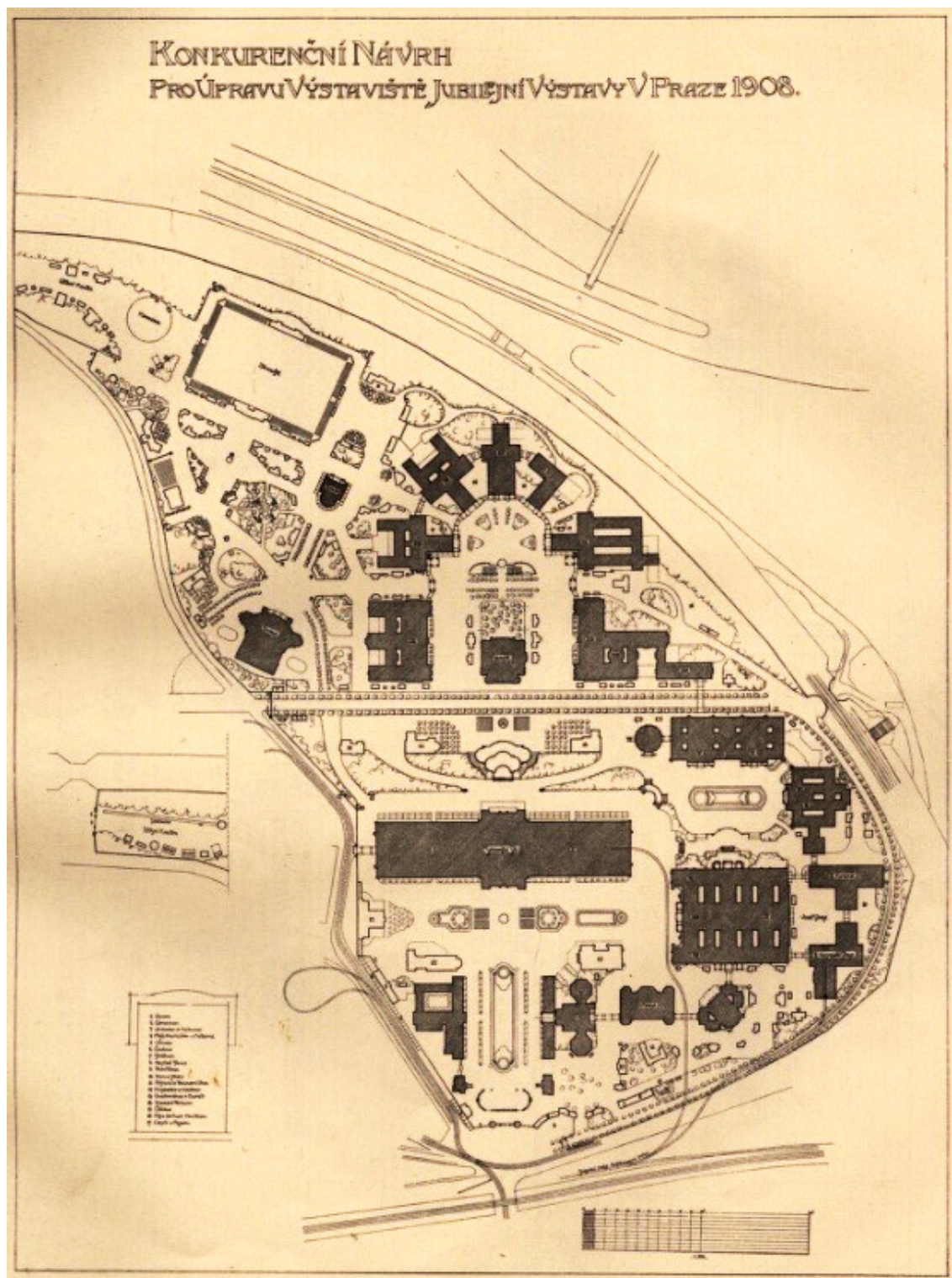
Obr. 15 Vítězný návrh prof. Rudolfa Kříženeckého pro úpravu výstaviště pro Jubilejní výstavu v Praze roku 1908. Zdroj: Architektonický obzor . Praha: Spolek architektů a inženýrů v Království českém, 7.1908, 12(12), obrazová příloha, obr. č.1. ISSN 1803-3350.
