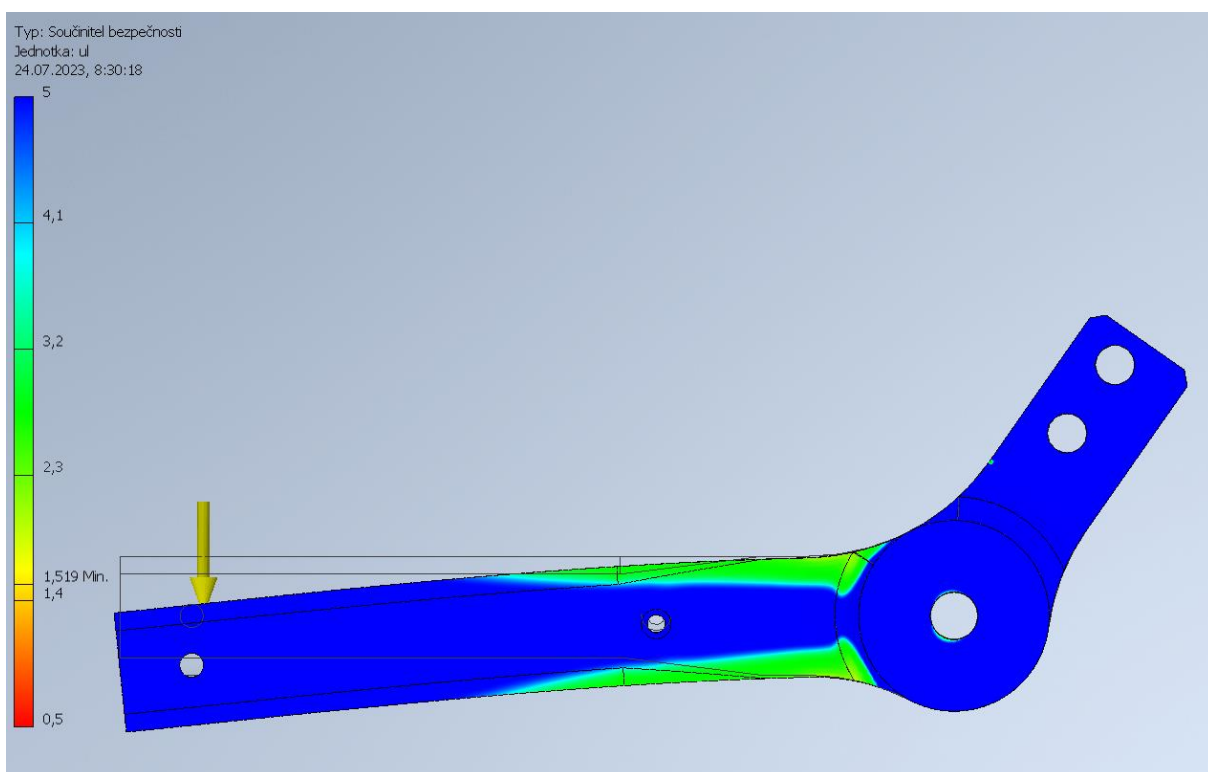
Obr. 10 Pevnostní analýza HTN-CF25 plné perimetry
