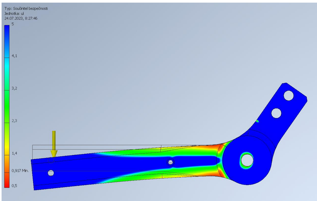
Obr. 6 Pevnostní analýza PETG-CF plné perimetry
