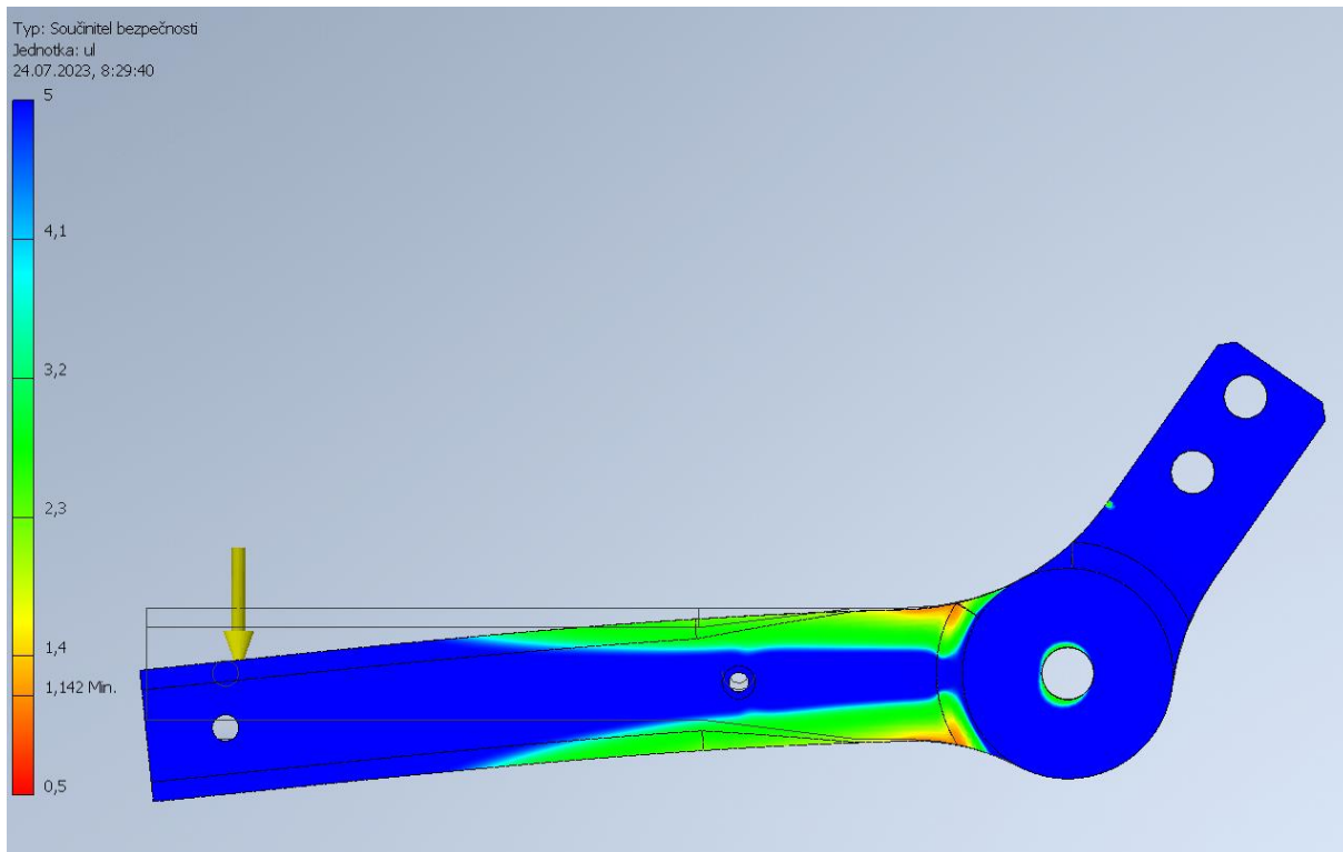
Obr. 9 Pevnostní analýza HTN-CF25 4 perimetry
