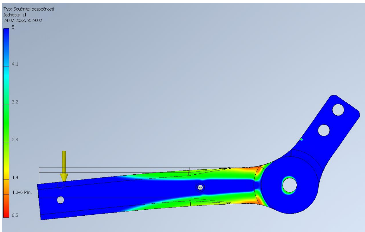
Obr. 8 Pevnostní analýza PA12-CF plné perimetry
