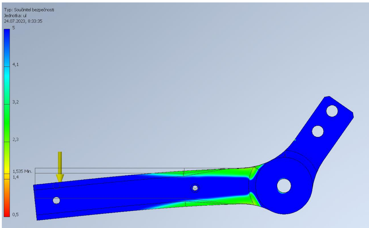
Obr. 14 Pevnostní analýza PA6-CF plné perimetry
