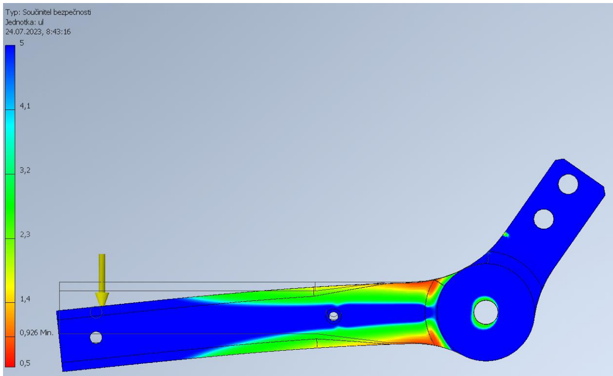
Obr. 1 Pevnostní analýza PETG 4 perimetry
