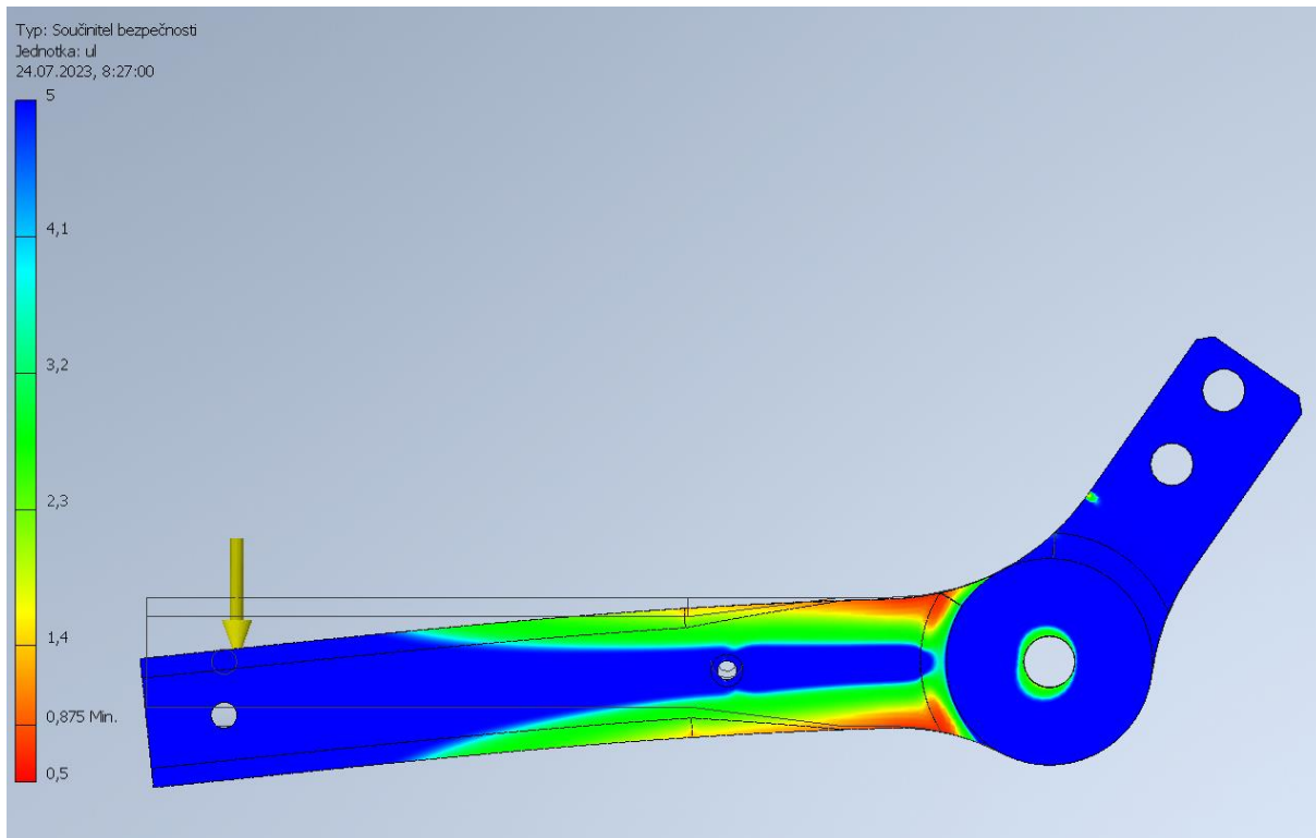
Obr. 5 Pevnostní analýza PETG-CF 4 perimetry
