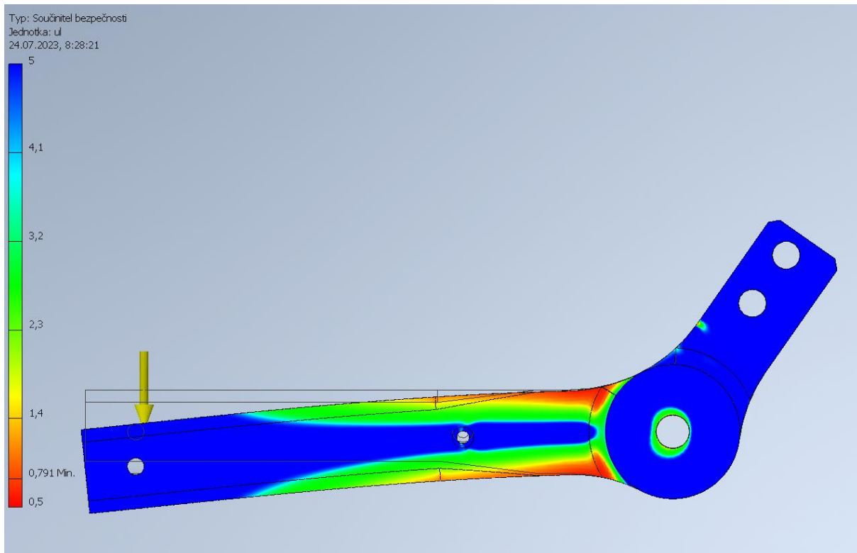
Obr. 7 Pevnostní analýza PA12-CF 4 perimetry
