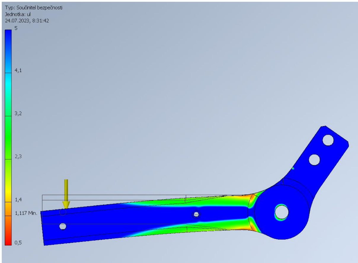
Obr. 11 Pevnostní analýza PC 4 perimetry
