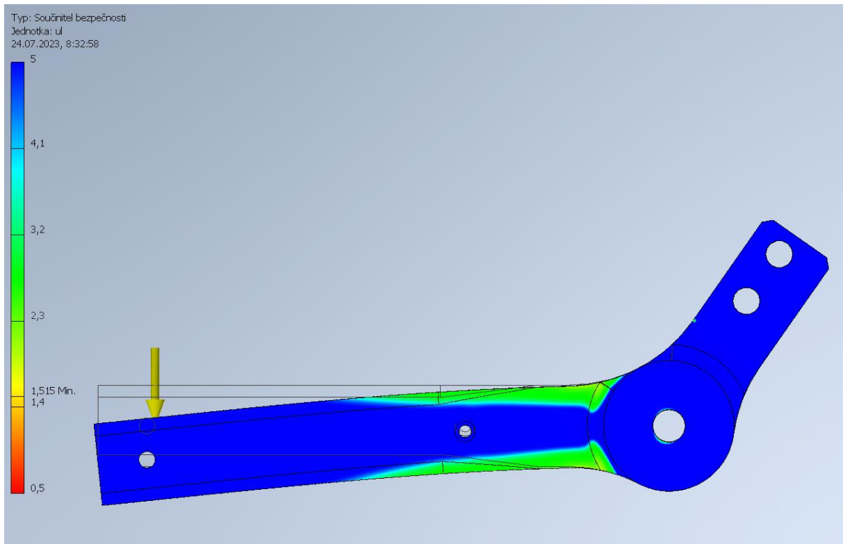
Obr. 13 Pevnostní analýza PA6-CF 4 perimetry
