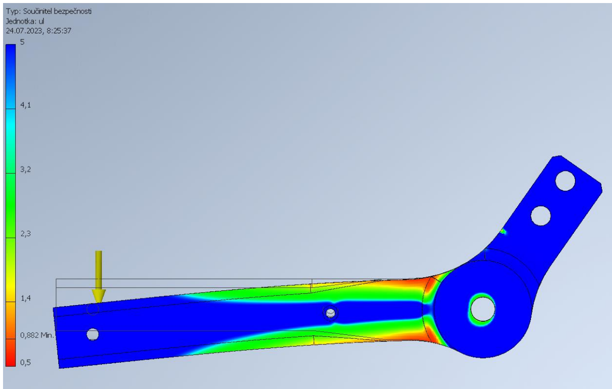
Obr. 3 Pevnostní analýza CPE HG100 4 perimetry
