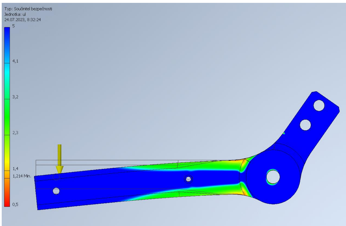
Obr. 12 Pevnostní analýza PC plné perimetry
