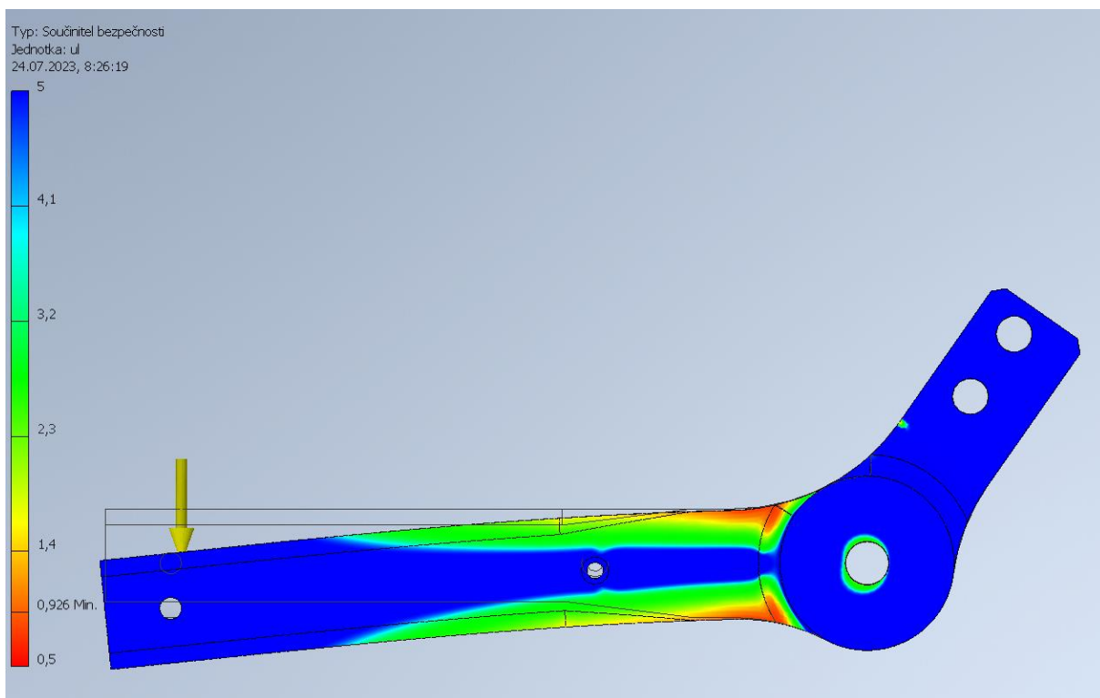
Obr. 4 Pevnostní analýza CPE HG100 plné perimetry
