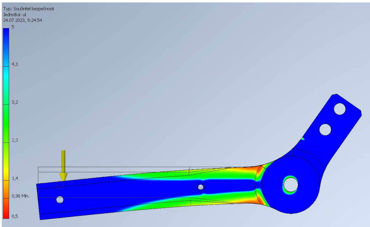
Obr. 2 Pevnostní analýza PETG plné perimetry
