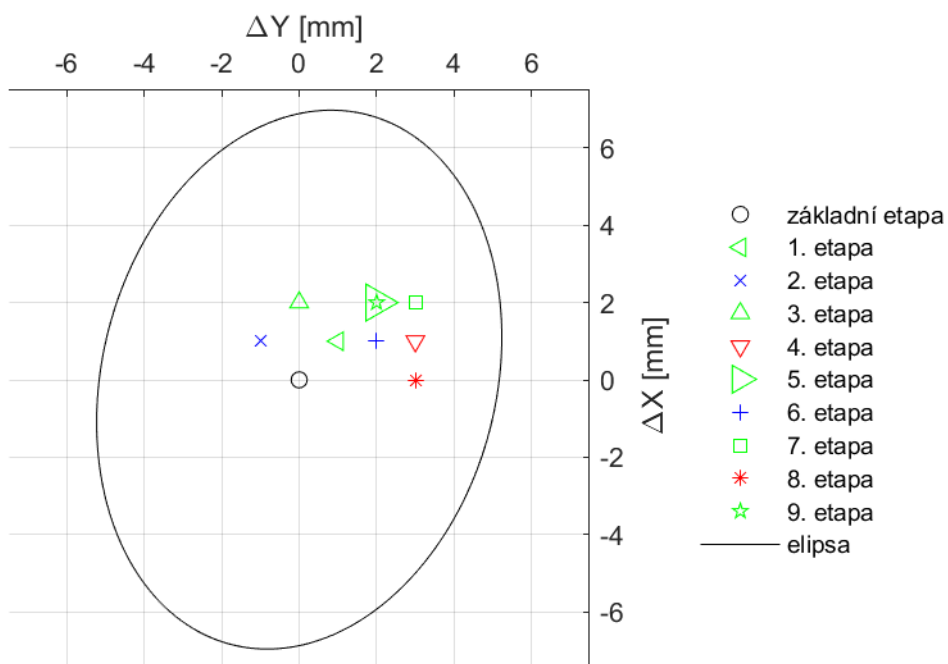
Poloha kontrolního bodu KB07
