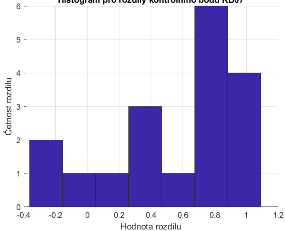
Histogram pro rozdíly kontrolního bodu KB07
