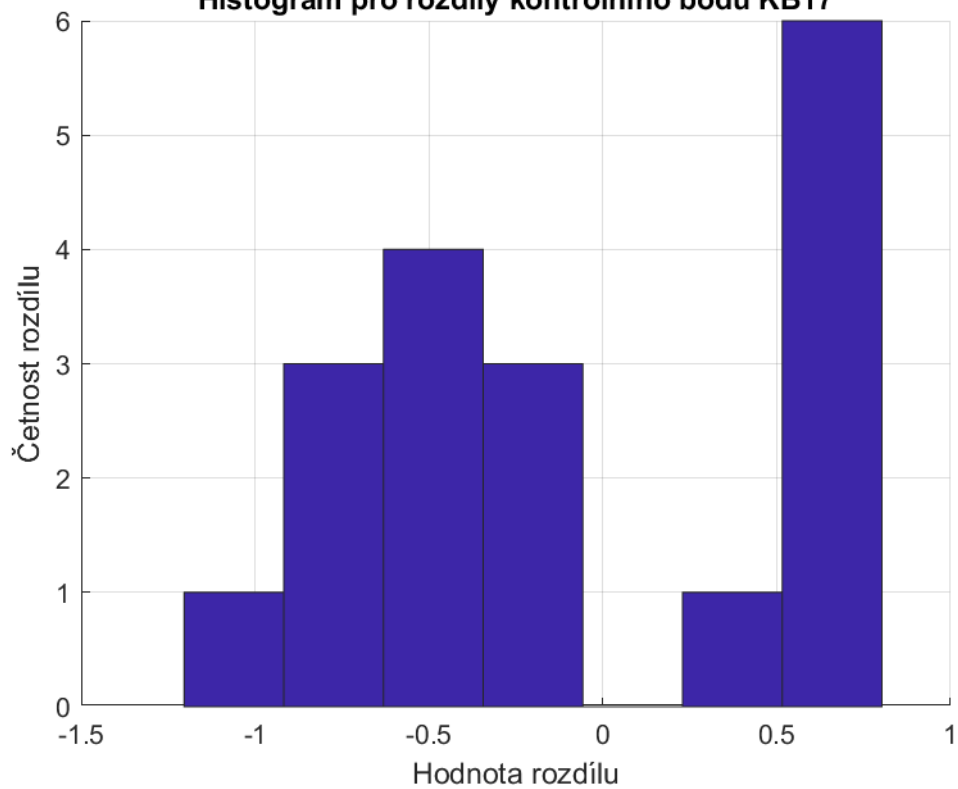
Histogram pro rozdíly kontrolního bodu KB17
