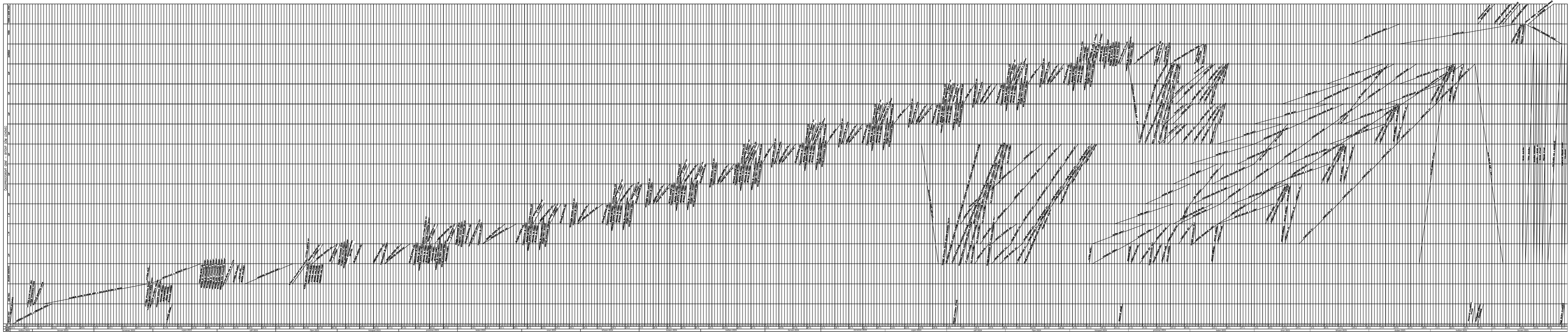
4.1 ČASOPROSTOROVÝ GRAF
