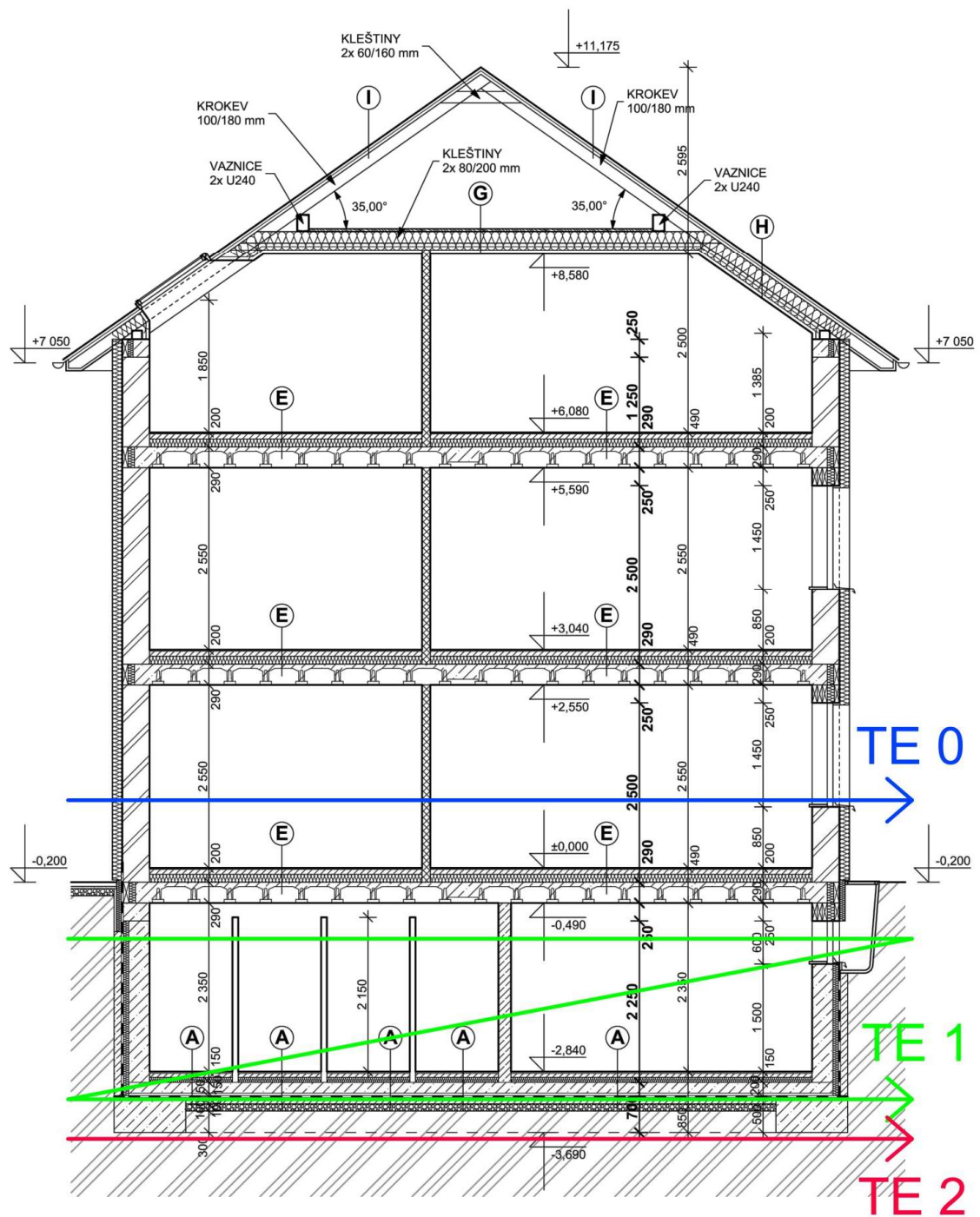
Obr. 1 - Schéma postupu výstavby 0., 1. a 2. TE
