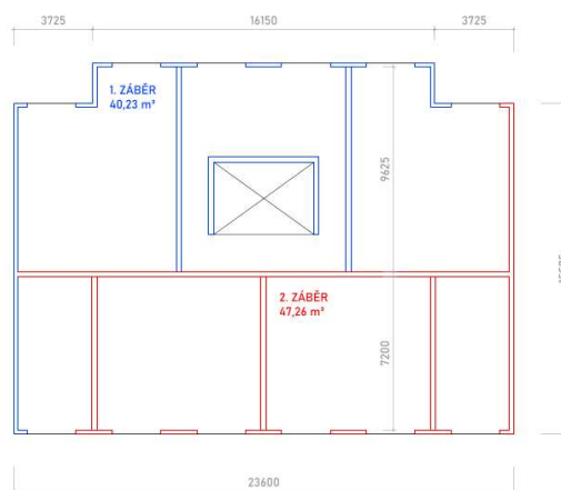
náčrt záběrů – svislé konstrukce
