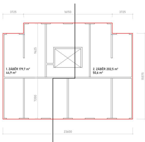
náčrt záběrů – vodorovné konstrukce
