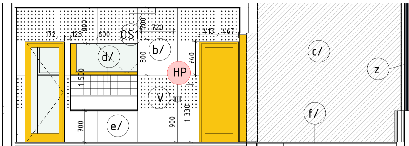
jižní stěna
