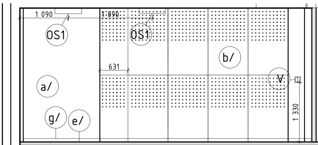
severní stěna
