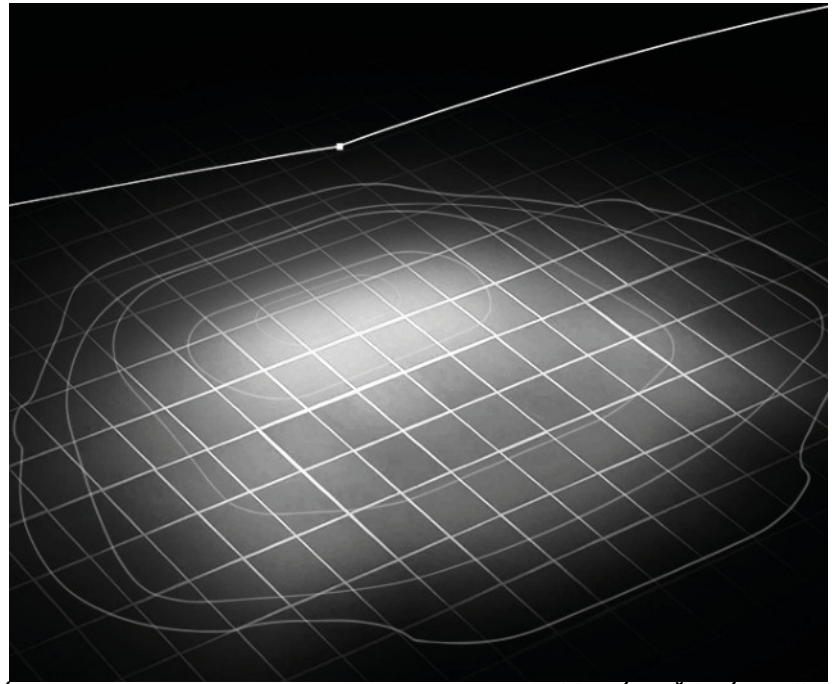
hlavní osvětlení - optika
