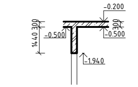
⑤ - ŘEZ NADPRAŽÍM DVEŘÍ
