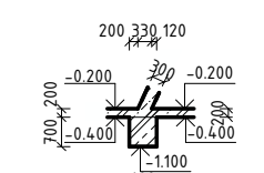
⑧ - ZÁKLAD ŠIKMÝCH STĚN VSTUPU
