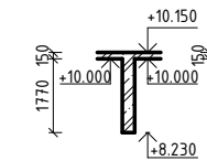
17 - NADPRAŽÍ DVEŘÍ technologických kabin
