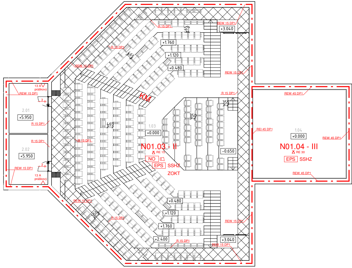
Púdorys 2NP - Požární bezpečnost
