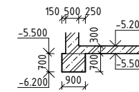
① - ZÁKLADY OBVODOVÝCH STĚN SUTERÉNU stěna tl. 500 mm
