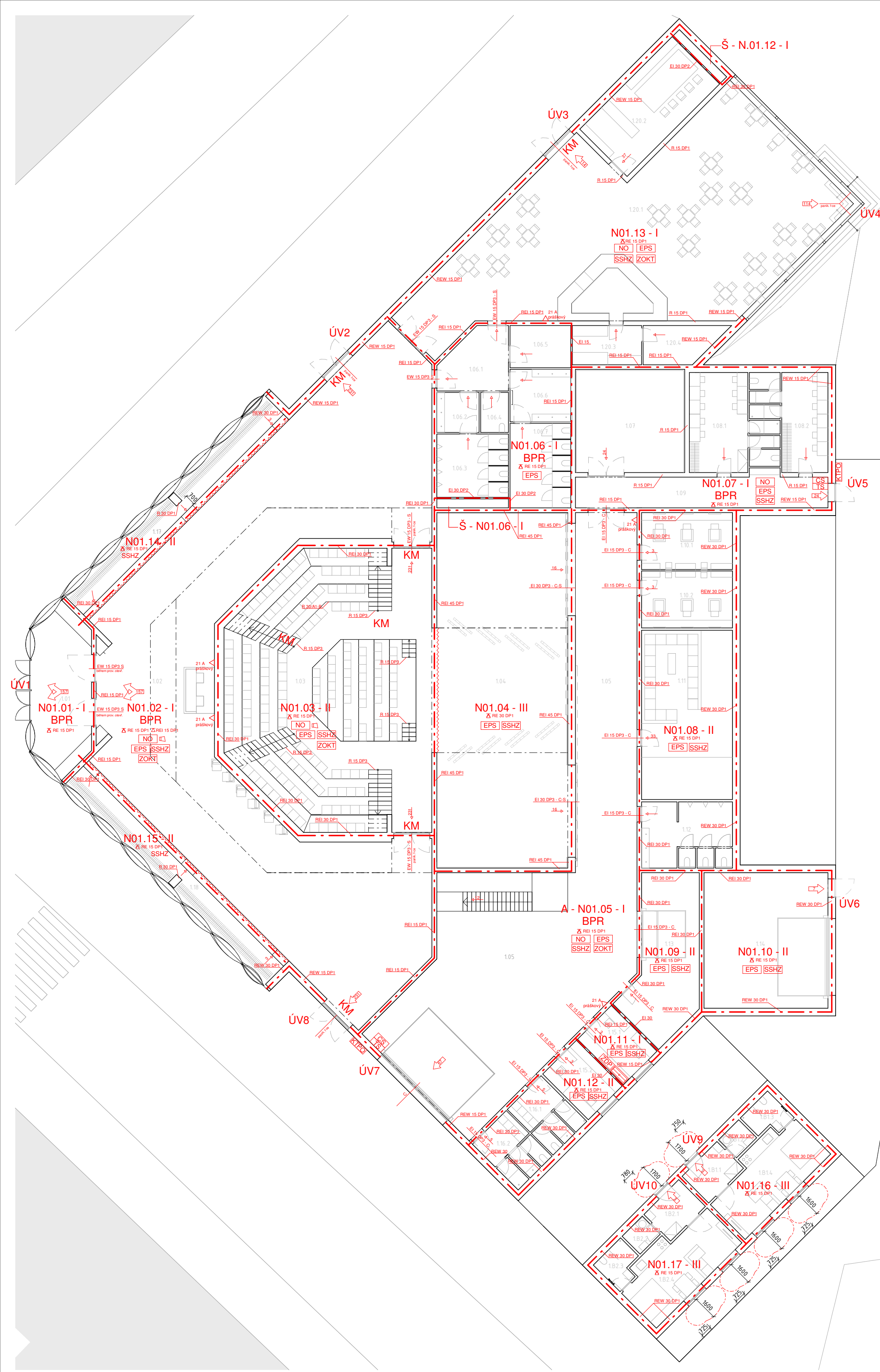
Púdorys 1NP - Požární bezpečnost
