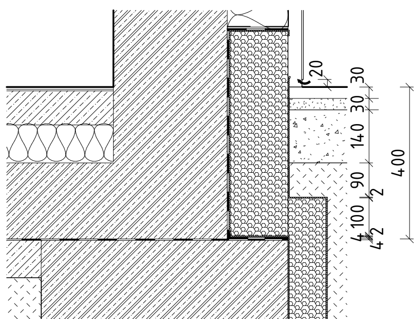
DET3 - detail soklu TOP
