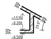
⑦ - NÁVAZNOST TRIBUNY NA DESKU 1NP
