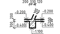
⑧ - ZÁKLAD ŠIKMÝCH STĚN VSTUPU
