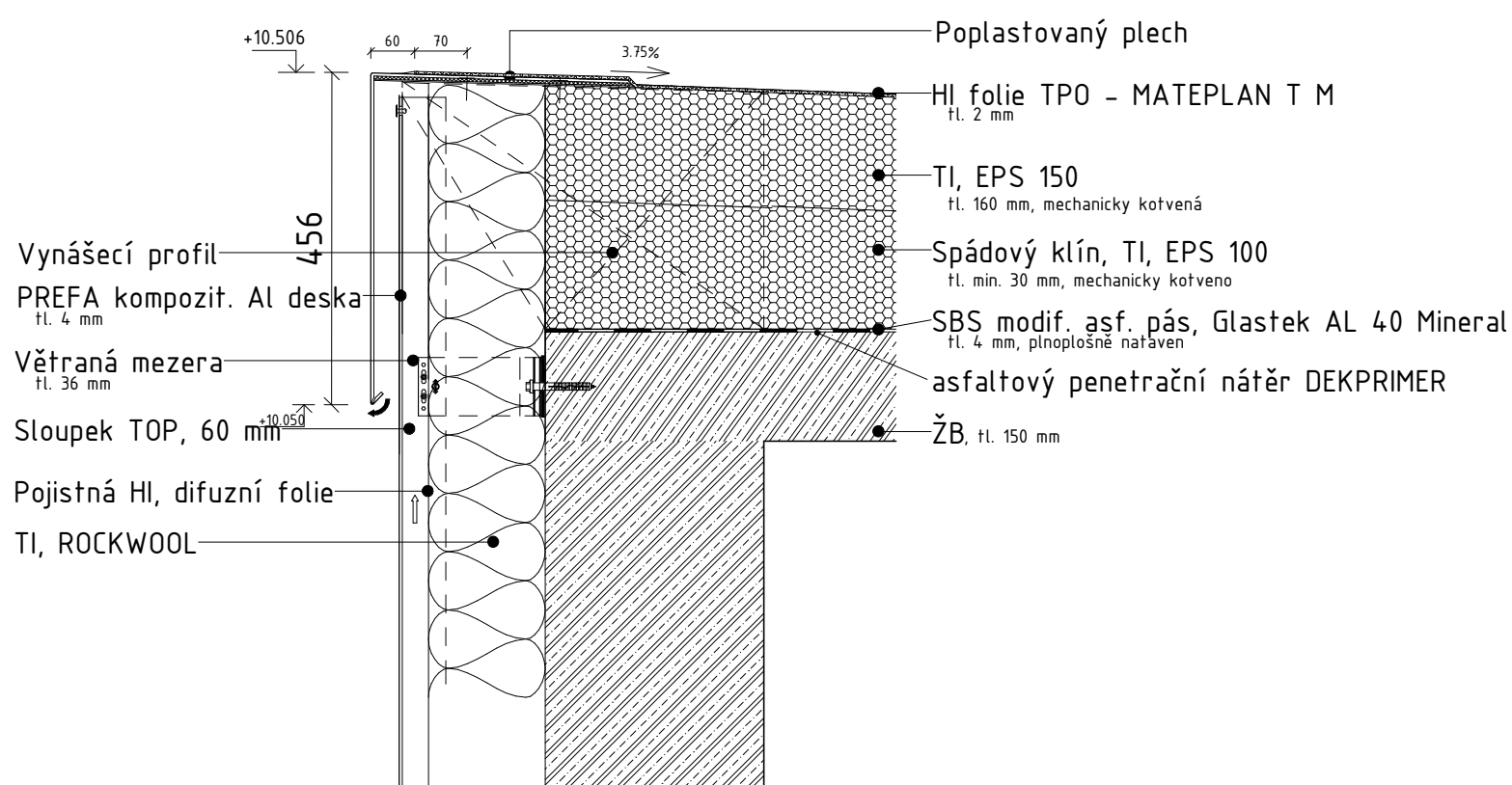
DET2 - detail atiky TOP
