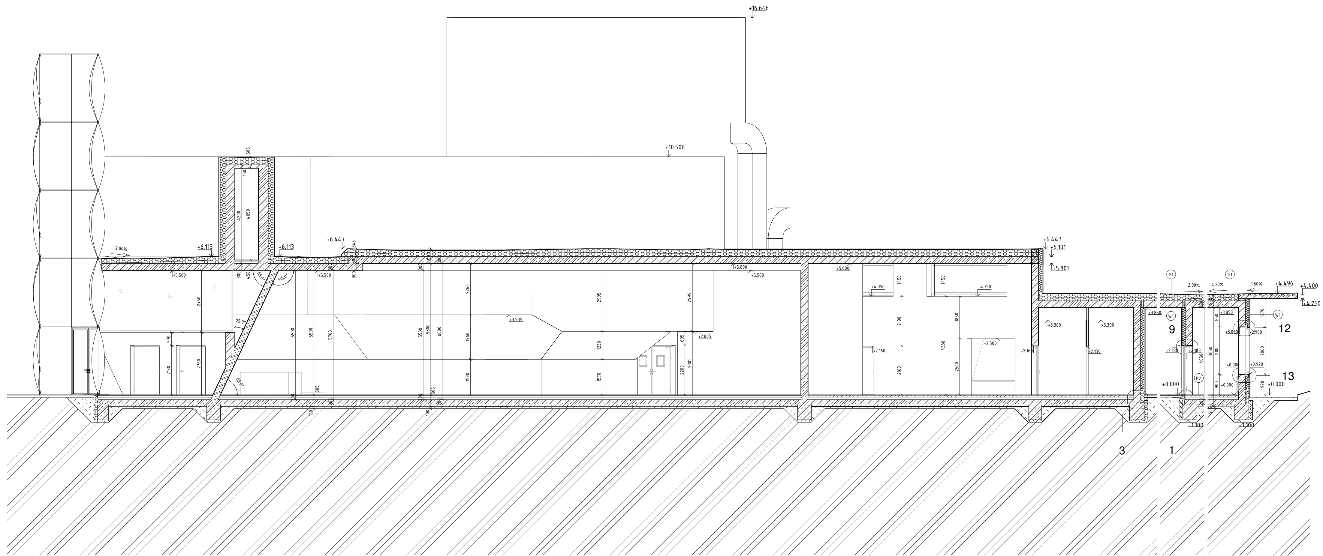
ŘEZ BB'
