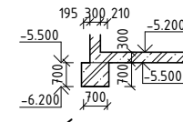
② - ZÁKLADY OBVODOVÝCH STĚN SUTERÉNU stěna tl. 300 mm
