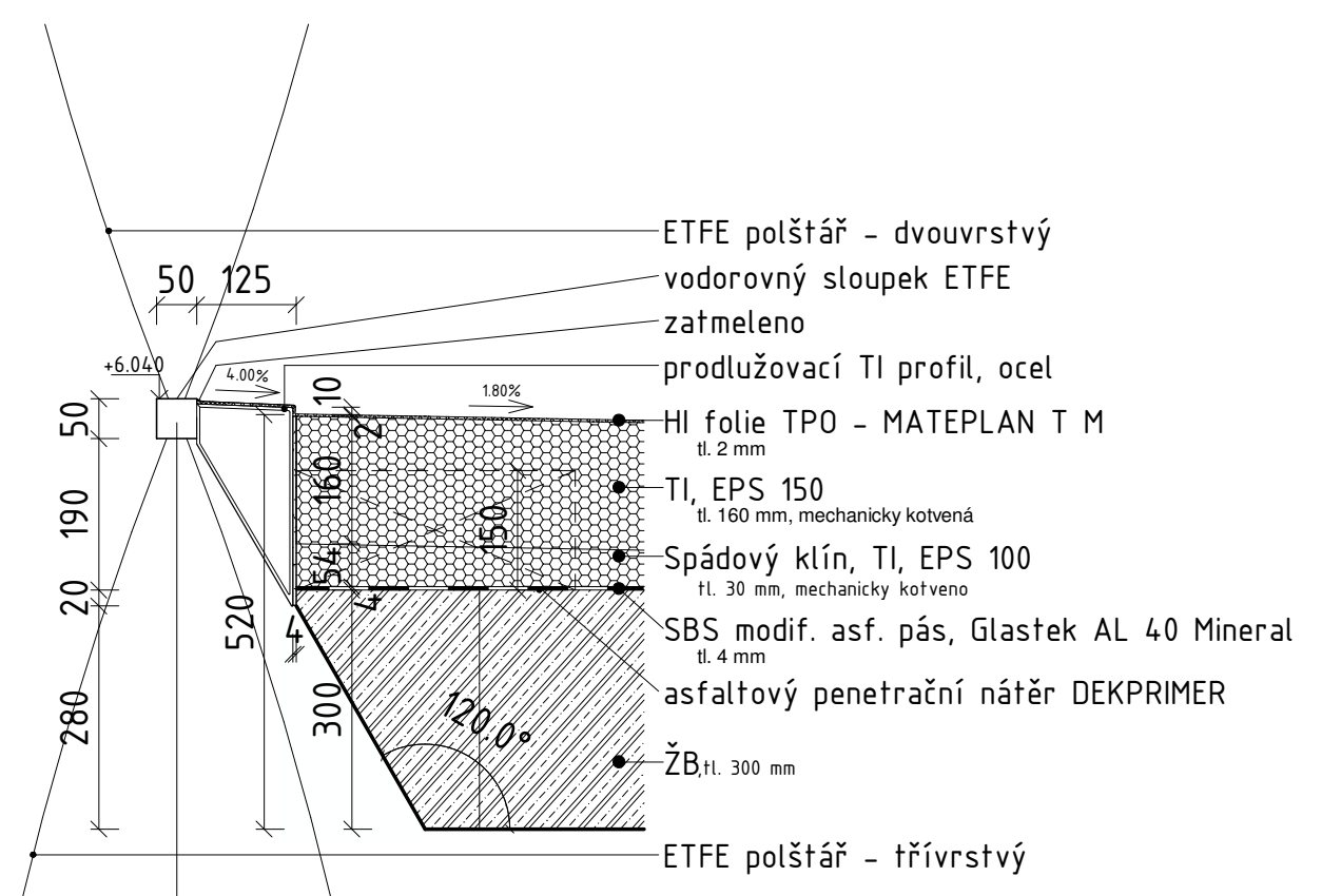
DET5 - přechod LOP
