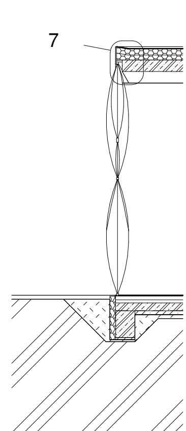
ŘEZ CC'
