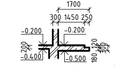
⑥ - OZUB OSAZENÍ PREFAB. SCHODIŠTĚ
