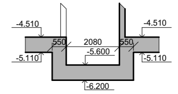
ŘEZ A-A'
