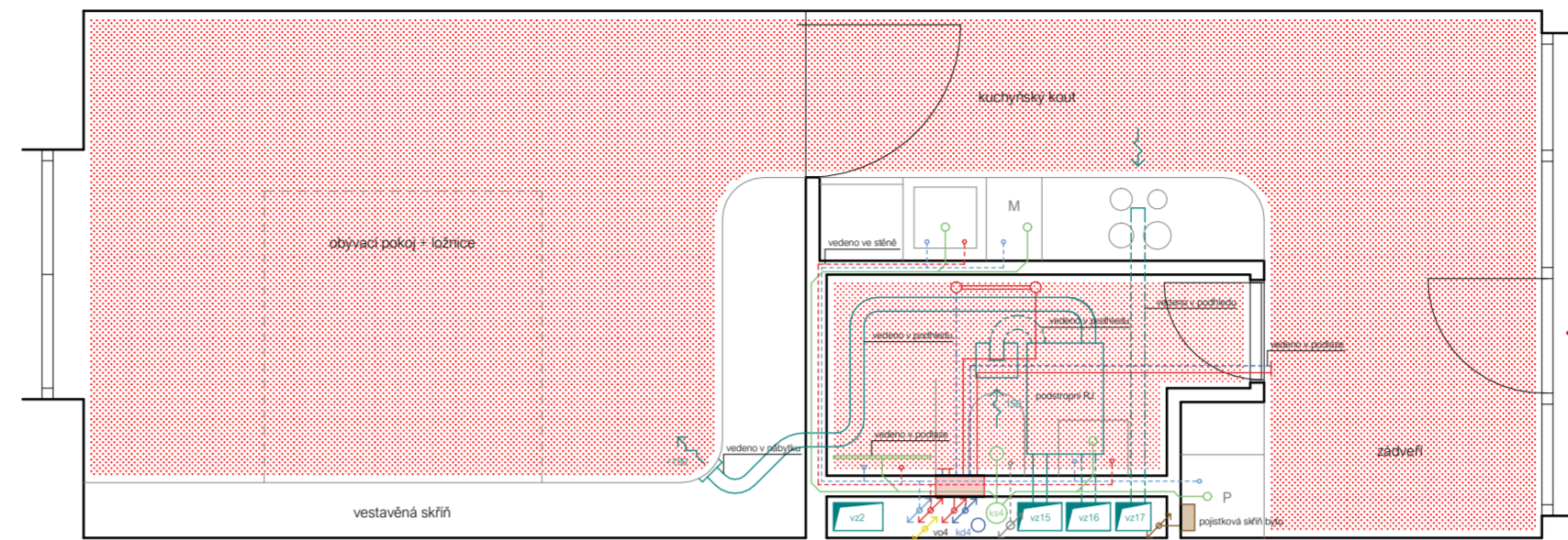
DETAIL BYTU 3.2 (1:50)
