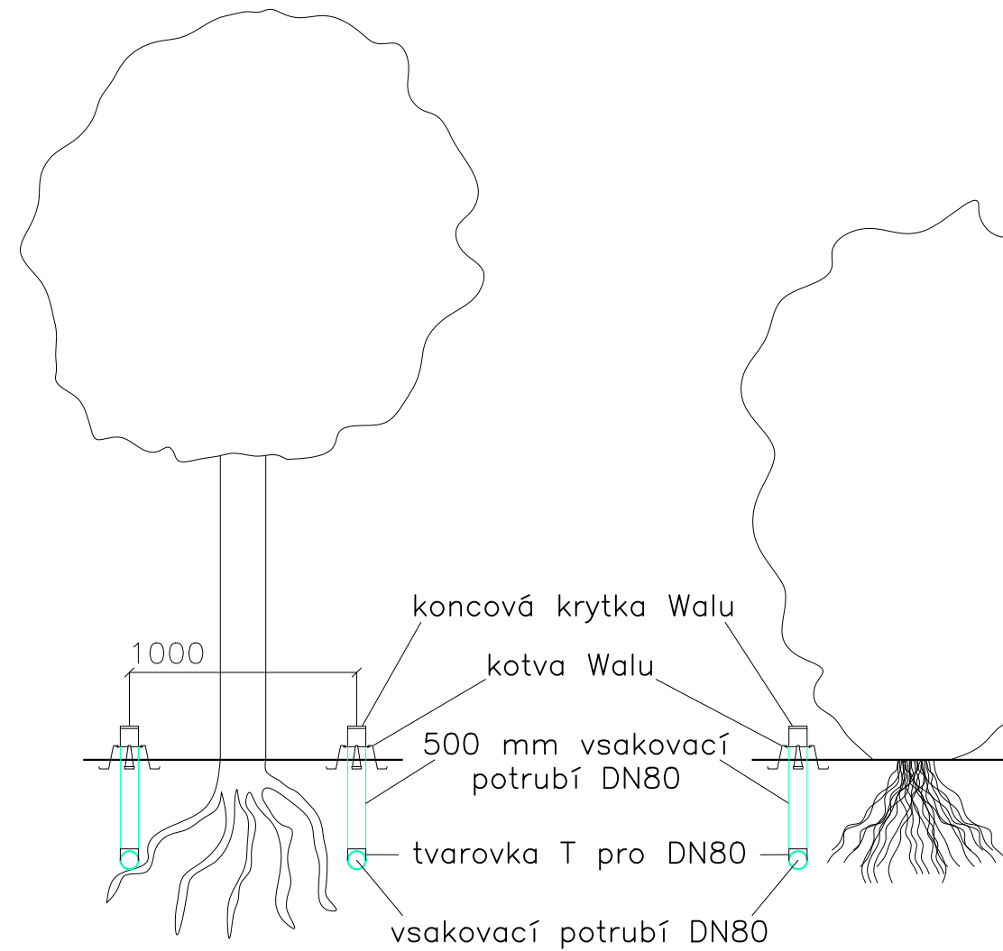
Vsakovací potrubí (ovocné stromy)
