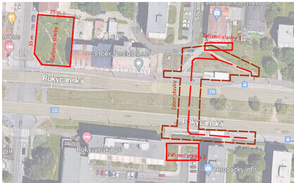
Obrázek 1 - Zařízení staveniště
