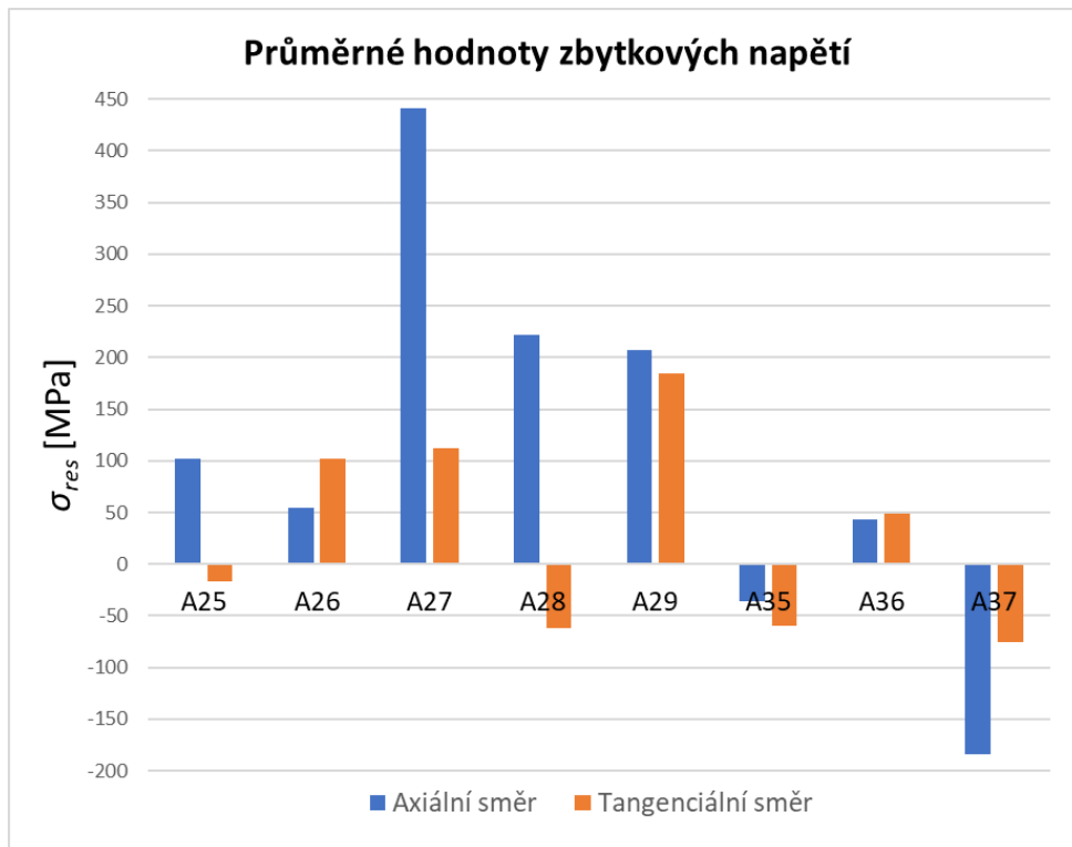
Obr. 15: Průměrné hodnoty zbytkových napětí
