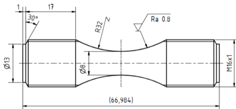
Obr. 13: Výkres vzorku
