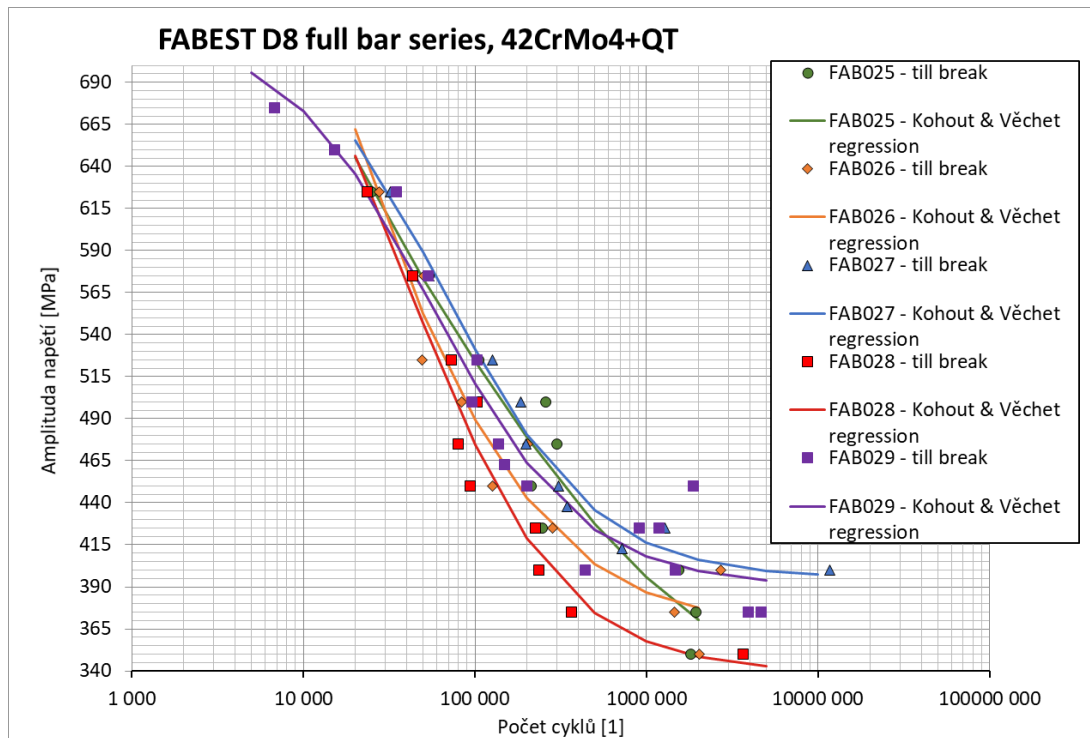
Obr. 16: Výsledky únavových experimentů, série A25-A29
