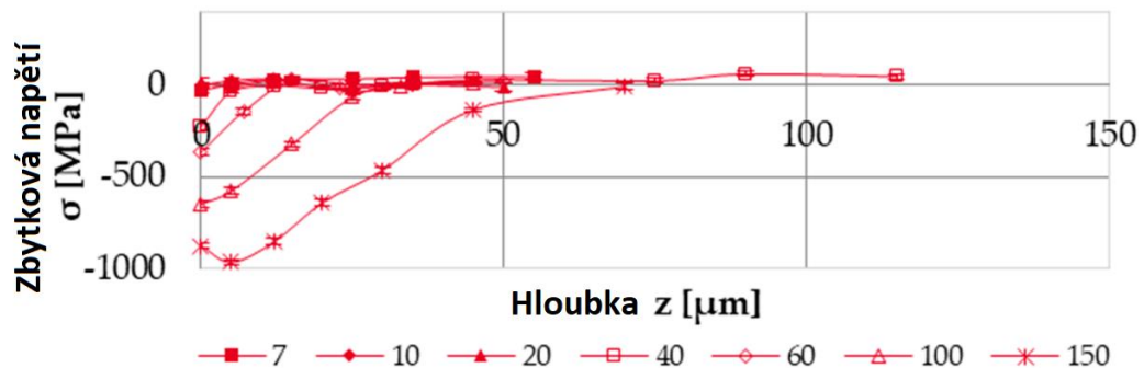
Obr. 9: Průběh zbytkových napětí po obrábění materiálu 42CrMo4 pro různé hloubky řezu, přeloženo z [18]
