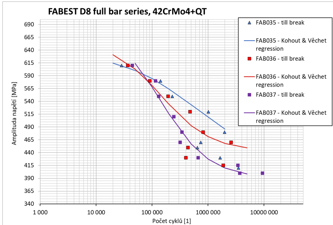
Obr. 17: Výsledky únavových experimentů, série A35-A37
