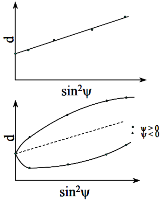
Obr. 7: Příklad regrese naměřených dat pomocí metody \sin^2 \psi [8]
