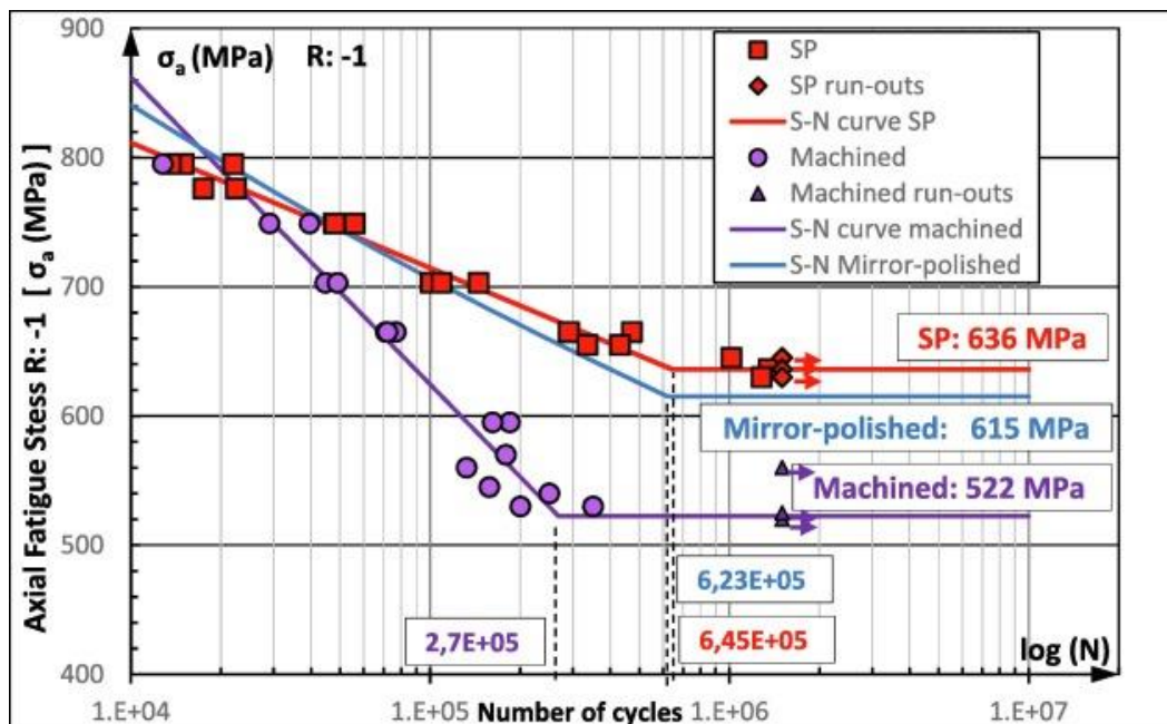
Obr. 12: Wöhlerovy křivky obrobených a kuličkových vzorků [11]
