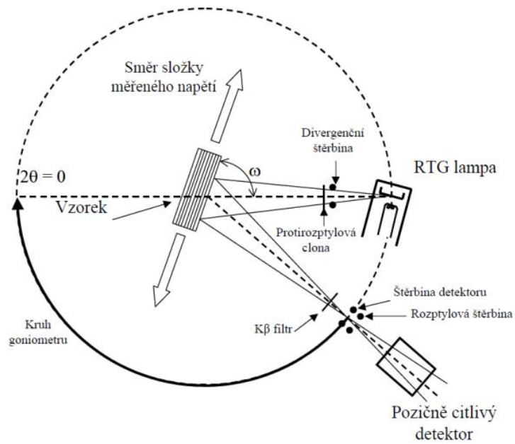
Obr. 8: Schéma laboratorního rentgenového difraktometru [7]
