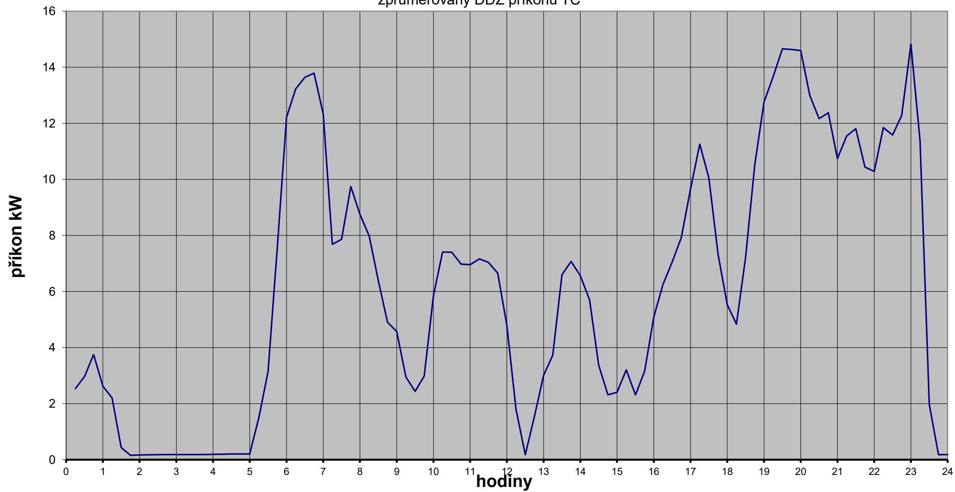
zprůměrovaný DDZ příkonu TČ
