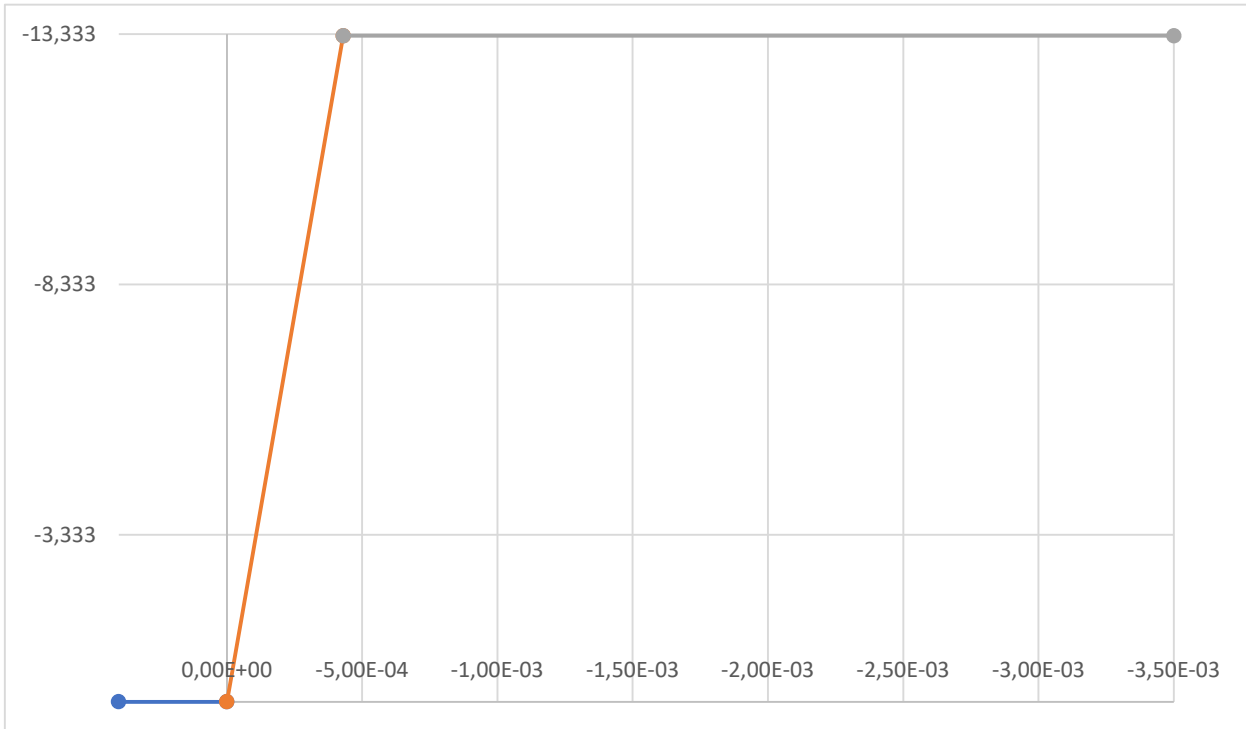
Pracovní diagram betonu C25/30
