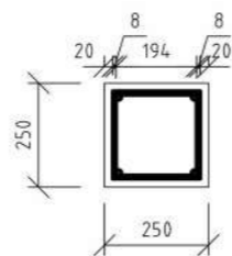
Řez A-A'
