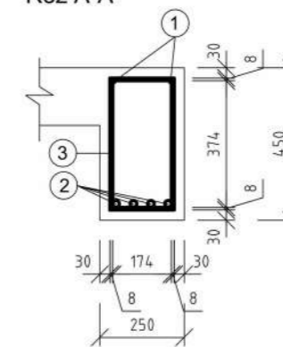
Řez A-A'
