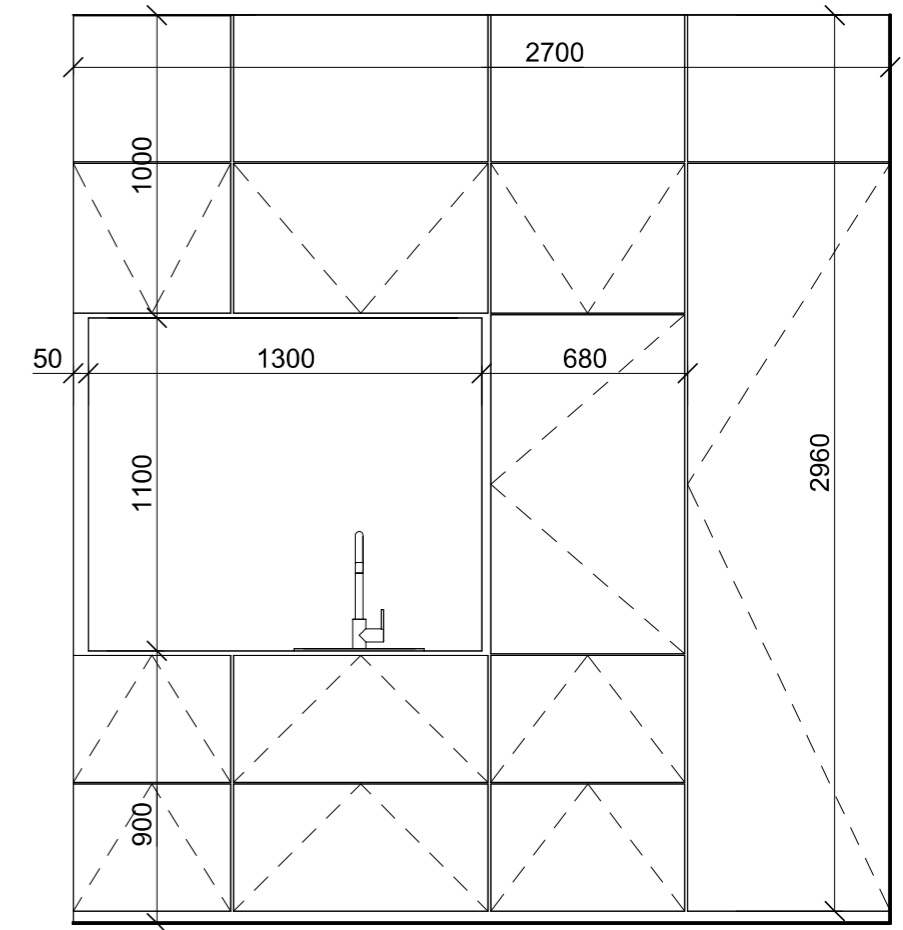
Atyp 2 1 : 25
