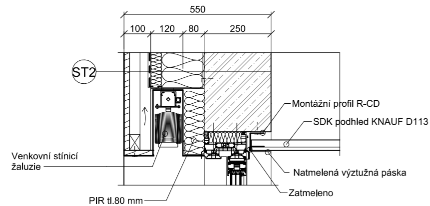
D4 1 : 10
