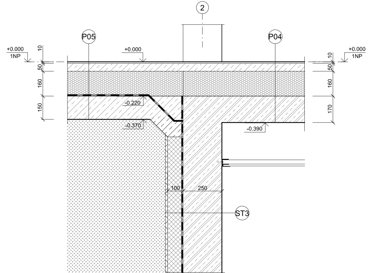
D5 1 : 10
