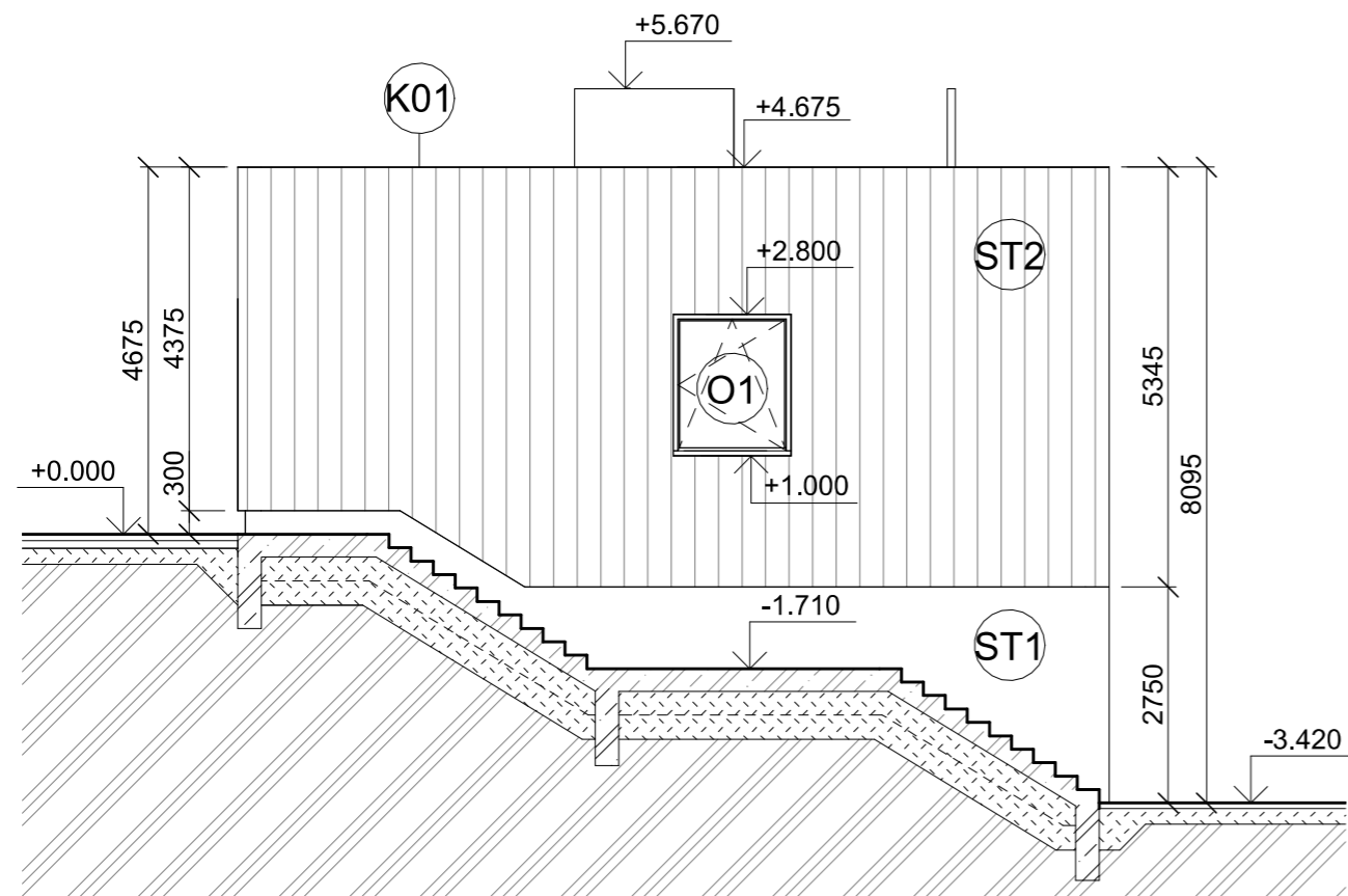
Východní pohled 1 : 100
