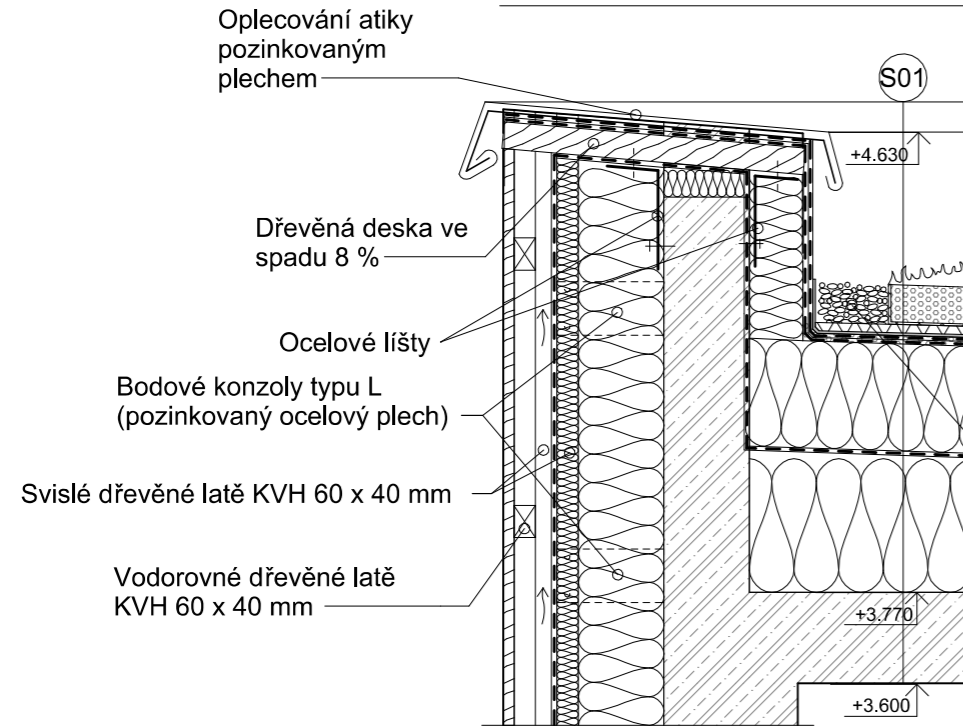
D3 1 : 10
