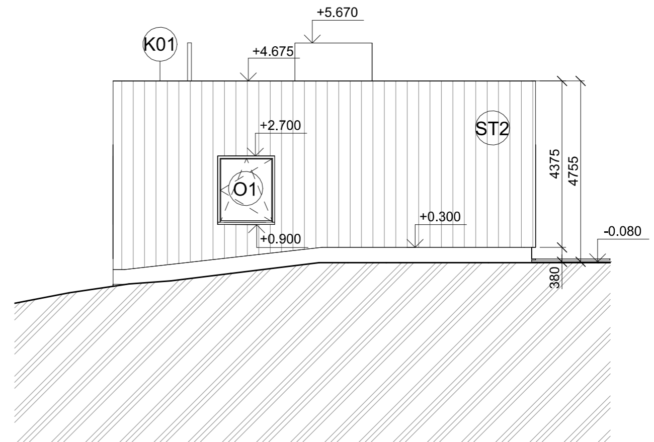
Zapadní pohled 1 : 100
