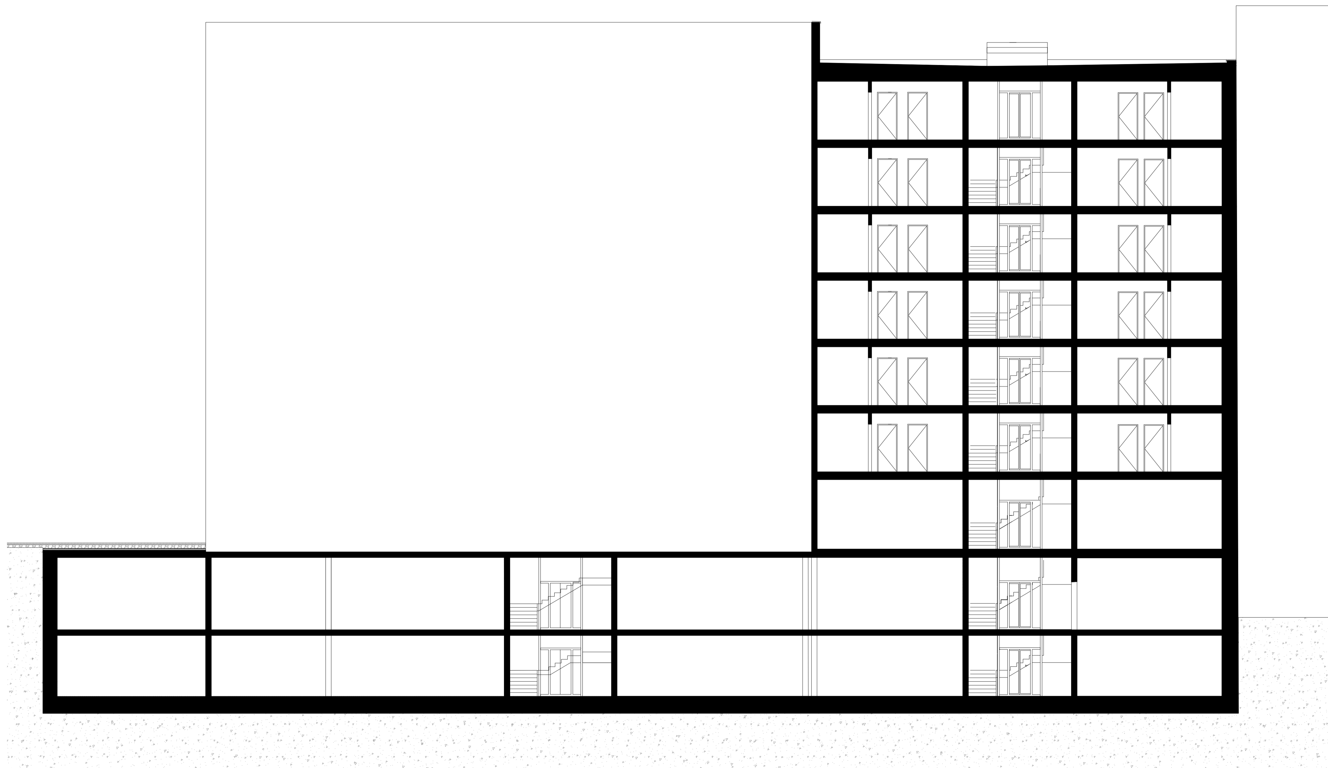
ŘEZ A-A'
