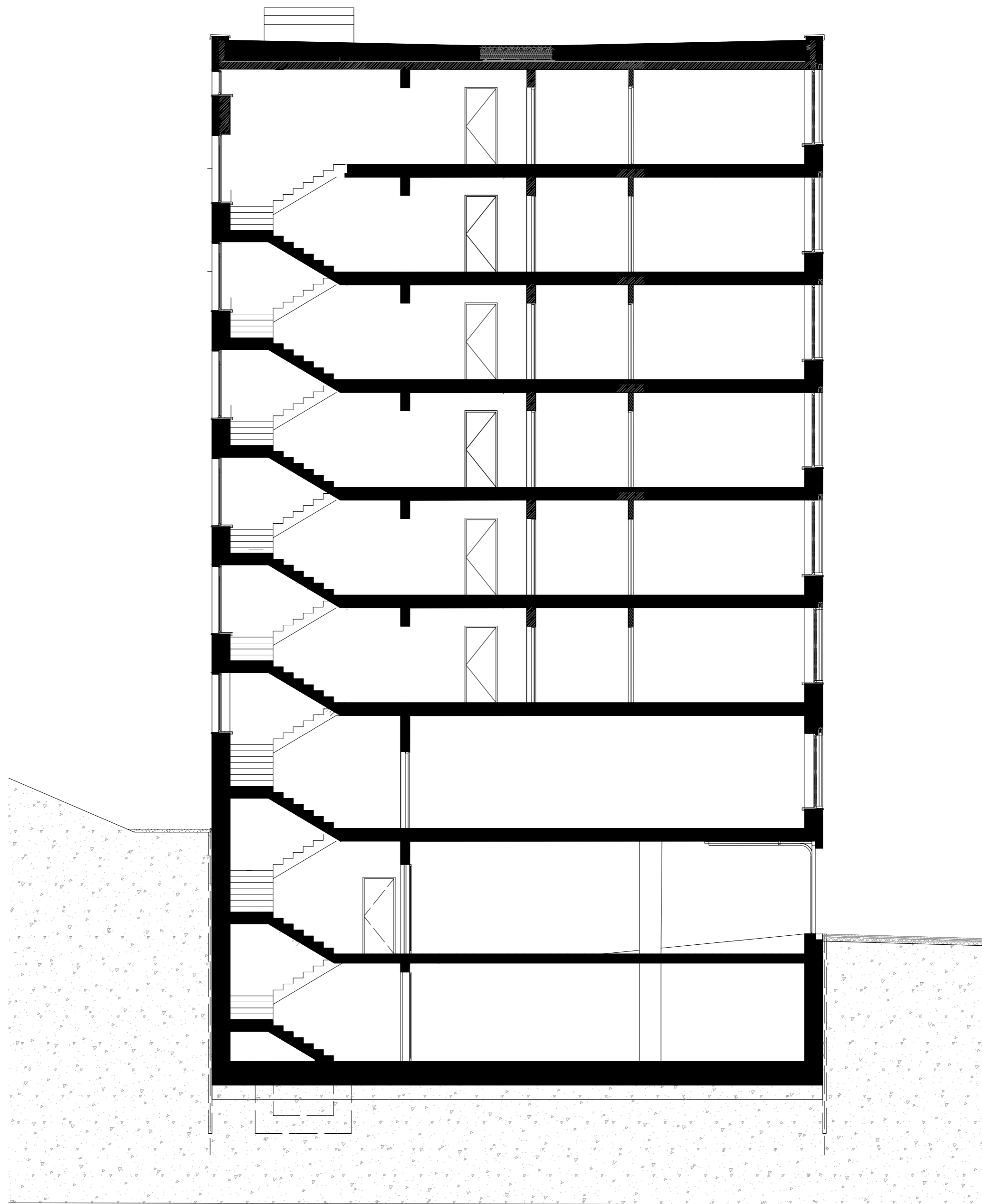
ŘEZ B-B'
