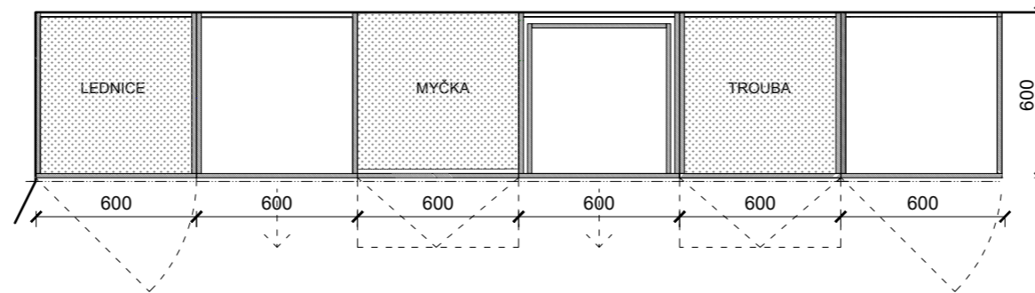
PŮDORYSNÝ ŘEZ
