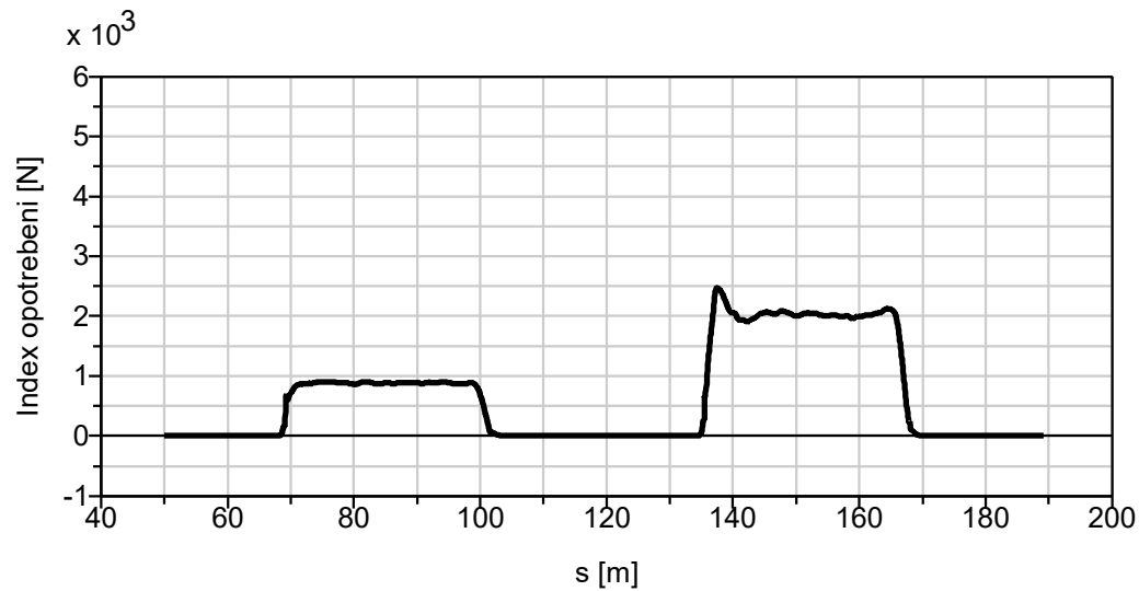
Leve zadni kolo
