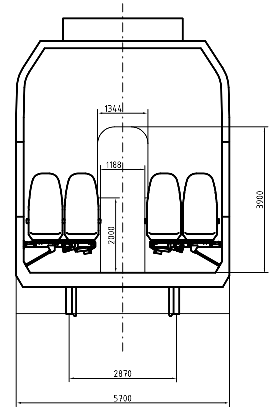
A - A (1 : 50)
