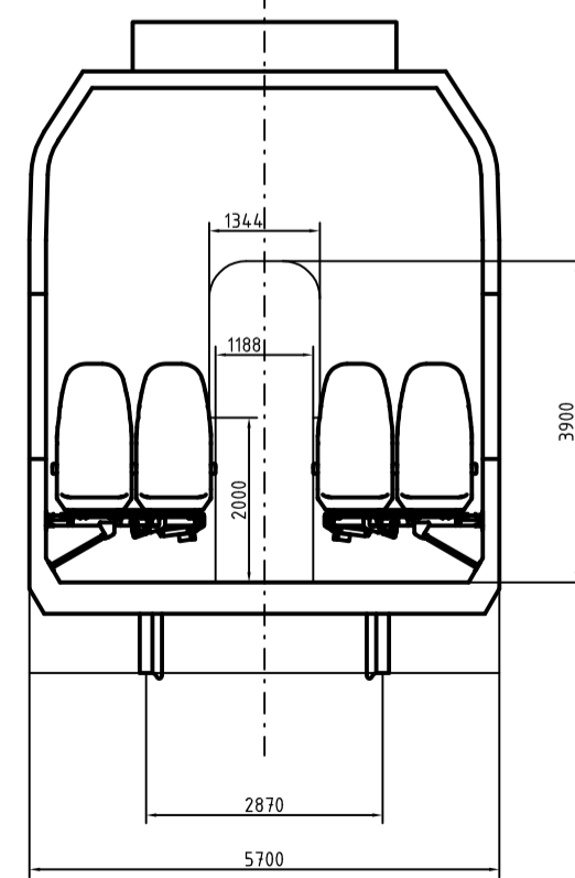
A - A (1 : 50)
