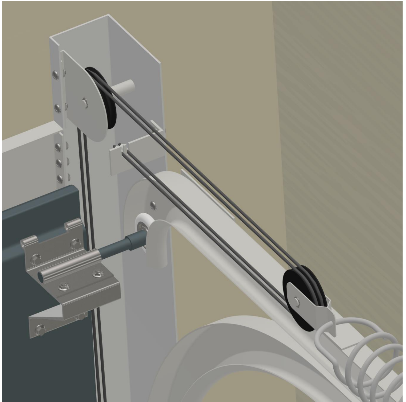
Příloha 2: Obrázek systému vyvážení vrat
