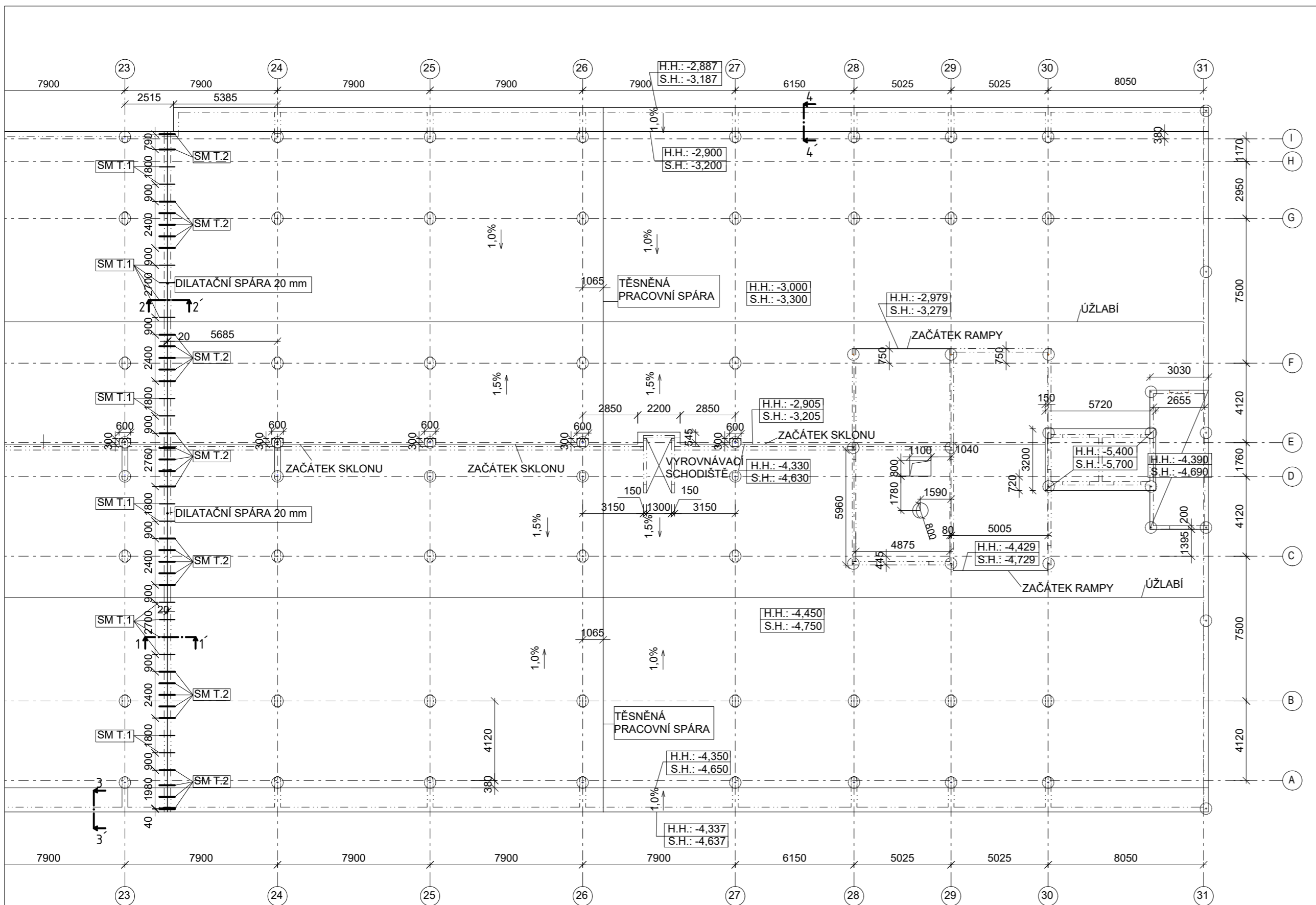
ZÁKLADOVÁ DESKA MĚŘITKO 1:200
