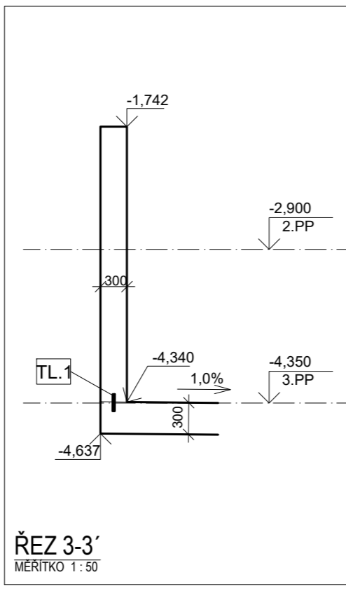
ŘEZ 3-3' MĚŘITKO 1:50
