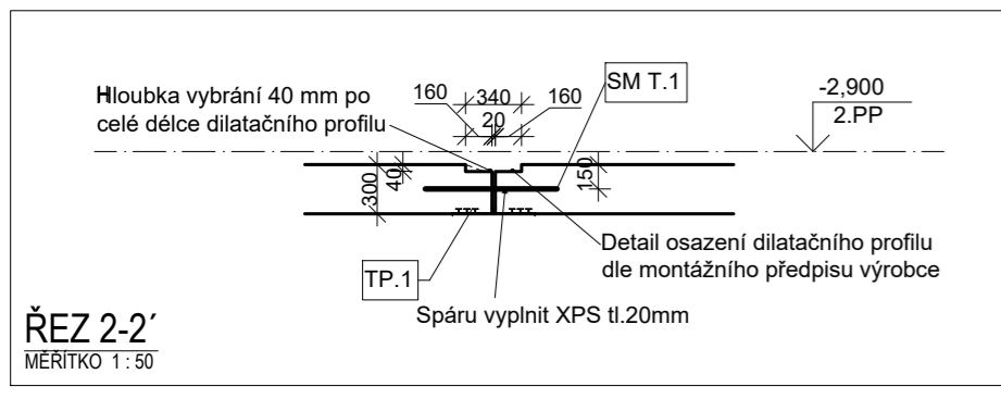
ŘEZ 2-2' MĚŘITKO 1:50
