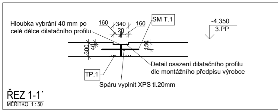
ŘEZ 1-1' MĚŘITKO 1:50
