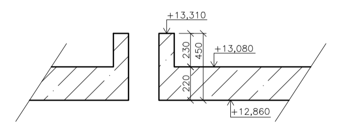
ŘEZ 1-1' M1:25
