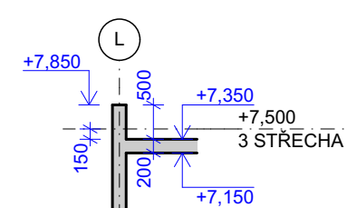
T1.2-3 ŘEZ 1:100
