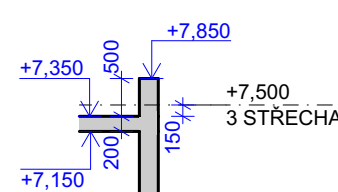
T1.2-2 ŘEZ 1:100
