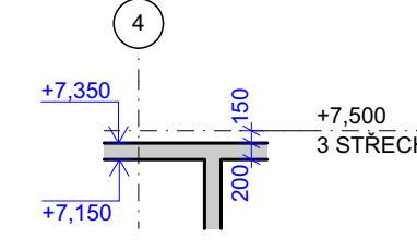
T1.2-6 ŘEZ 1:100
