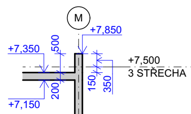
T1.2-1 ŘEZ 1:100
