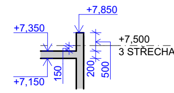
T1.2-4 ŘEZ 1:100
