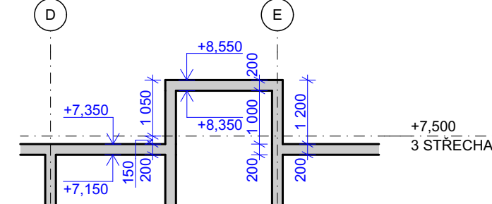
T1.2-5 ŘEZ 1:100
