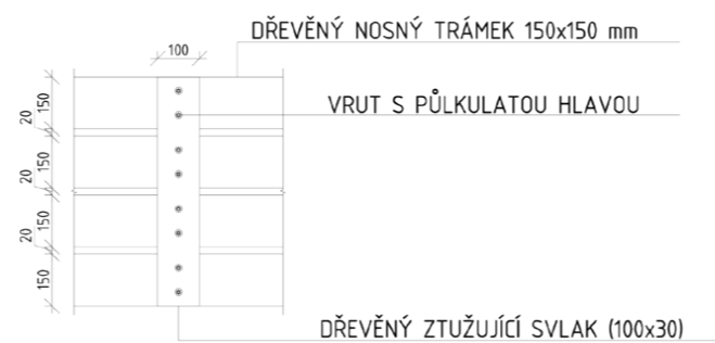
DETAIL SPOJENÍ TRÁMKŮ (SPODNÍ POHLED)
