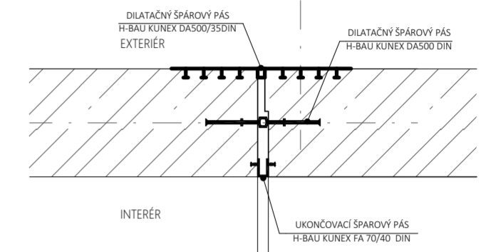
Detail dilatácie bielej väne M1:15
