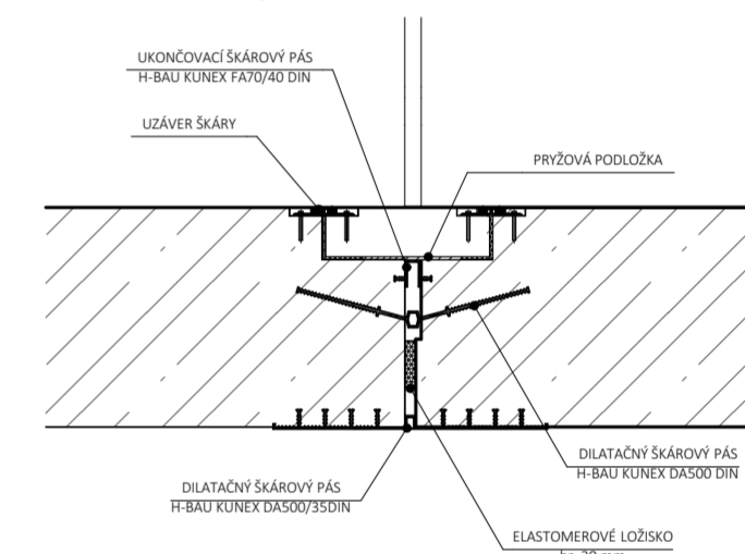
Detail dilatácie bielej väne M1:15
