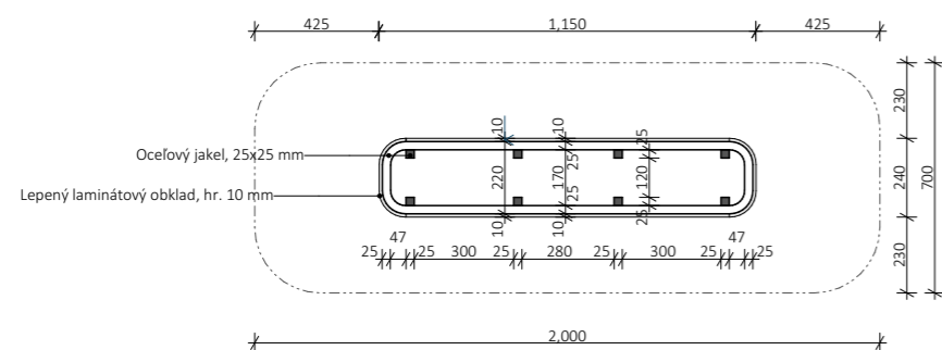
Vodorovný rez podstavou lehátka
