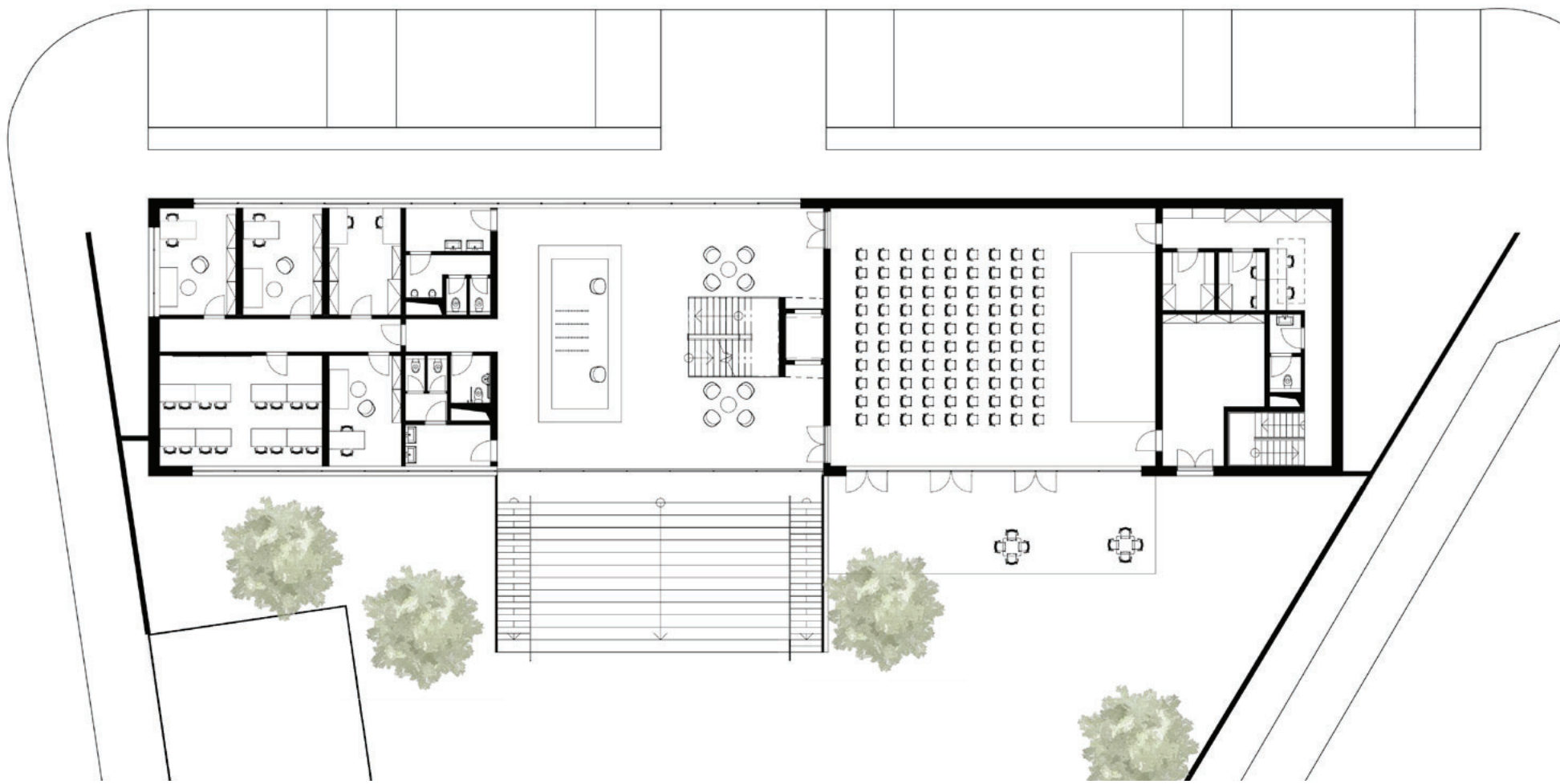
PŪDORYS 1. PATRA
