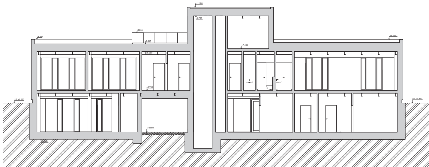
ŘEZ PODÉLNÝ
