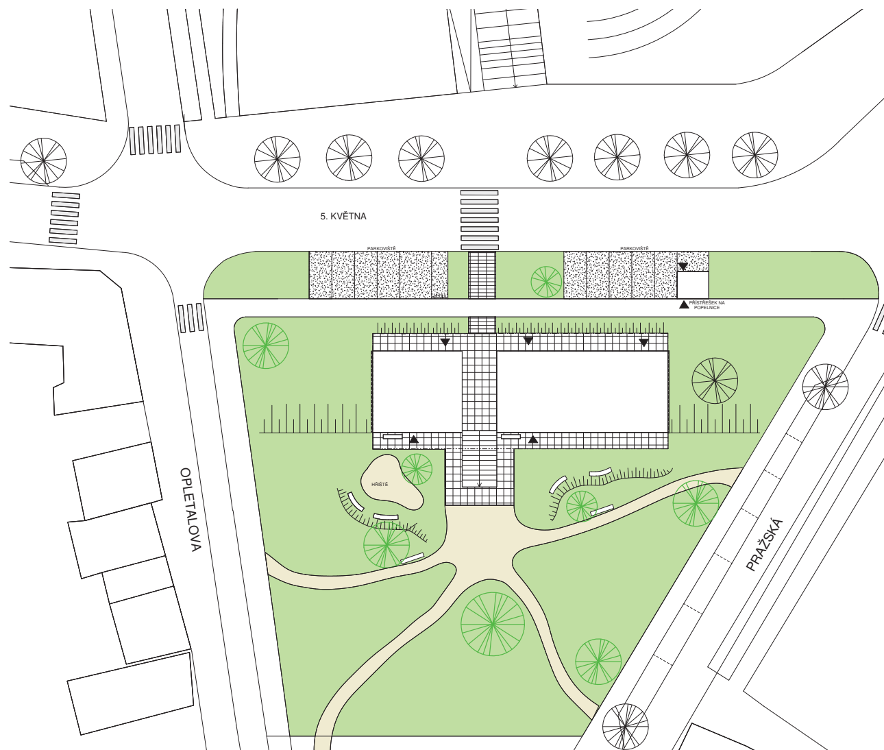
SITUACE
