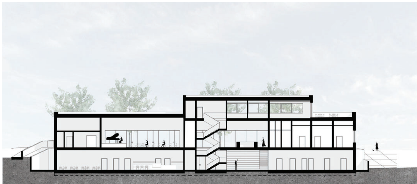
PODÉLNÝ ŘEZ
