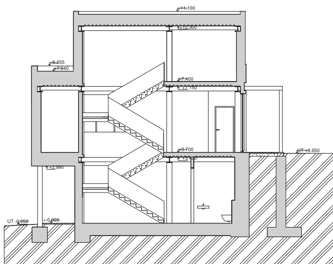
ŘEZ PŘÍČNÝ
