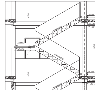
ŘEZ SCHODIŠTĚVÝM RAMENEM 2.NP A-A'
