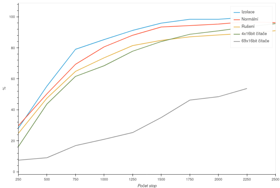
■ Obrázek 6.1 Úspěšnost korelační odběrové analýzy na FPGA
