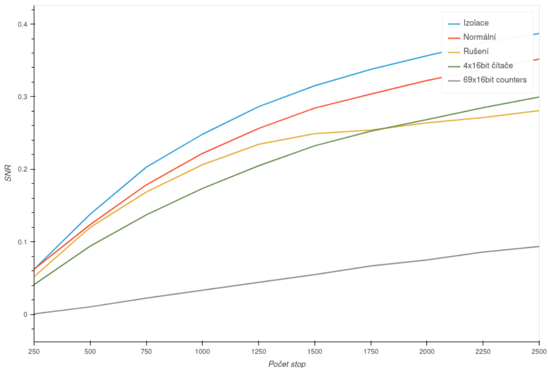
■ Obrázek 6.2 Odstup signálu od šumu na FPGA
