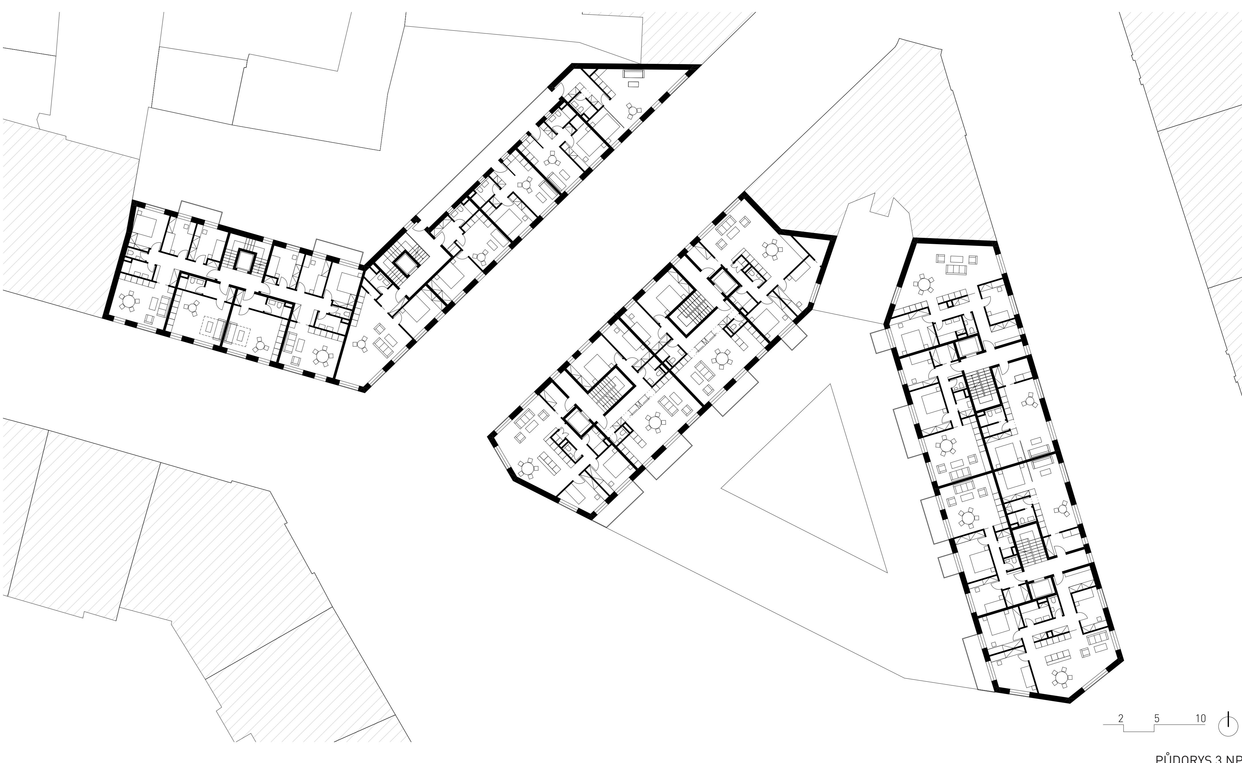
PŮDORYS 3.NP
