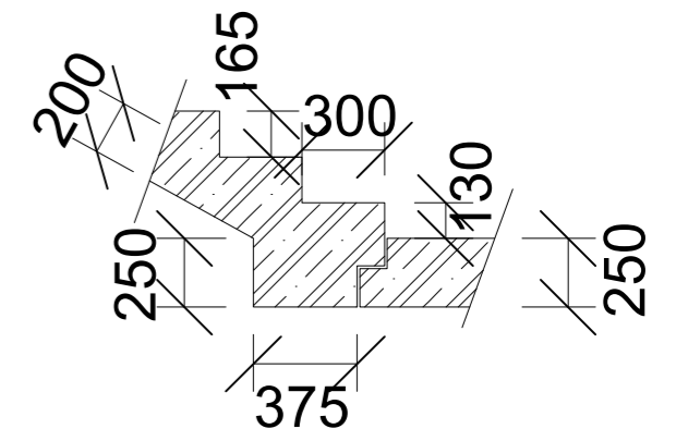
DETAIL NÁVAZNOSTI PREFABRIKOVANÉHO SCHODIŠŤOVÉHO RAMENE NA STROPNÍ DESKU, M1:30
